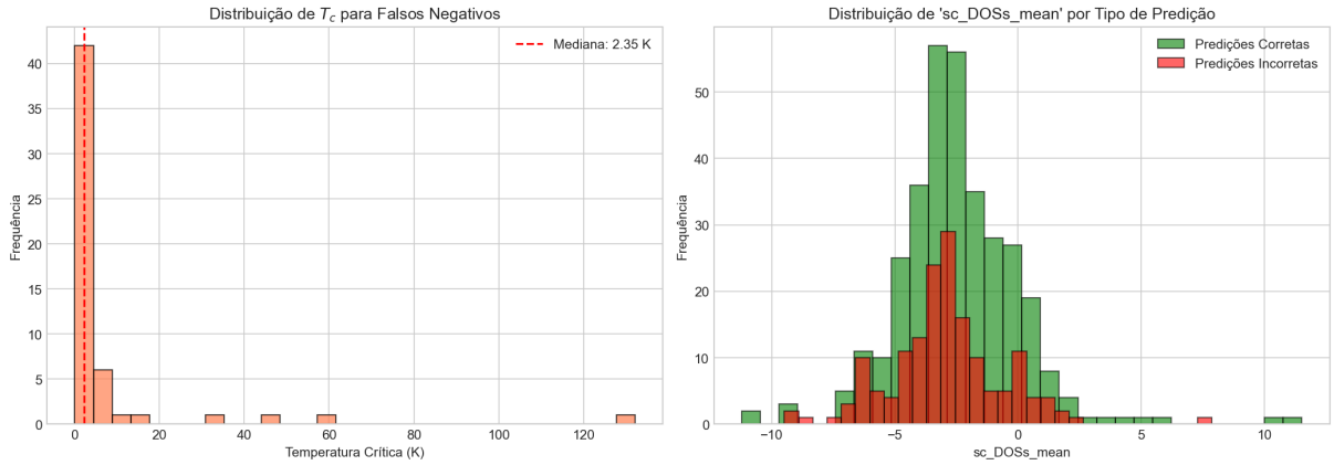
Figura 5.11: Análise de erro do modelo Random Forest. À esquerda, a distribuição de T_c para os Falsos Negativos. À direita, a distribuição da feature sc_DOSs_mean para predições corretas e incorretas.
