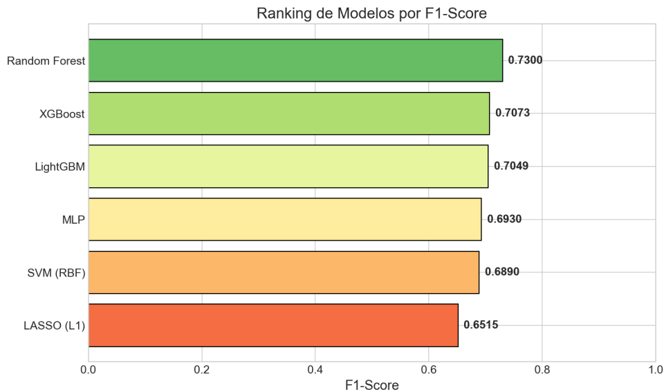
Figura 5.16: Ranking dos modelos com base no F1-Score no conjunto de teste. O Random Forest lidera, seguido de perto pelo XGBoost e LightGBM.
