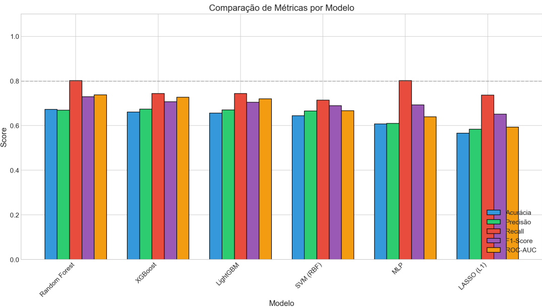
Figura 5.2: Comparação visual das métricas de desempenho para cada modelo. O Random Forest se destaca, especialmente em F1-Score e ROC-AUC.
