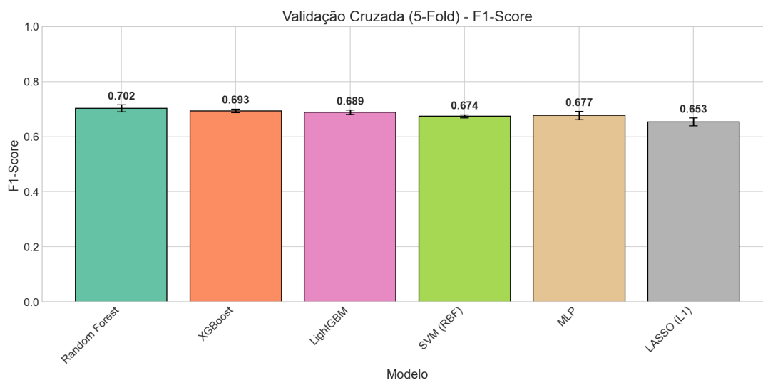
Figura 5.12: Resultados do F1-Score médio obtido com validação cruzada de 5 folds. As barras de erro representam o desvio padrão.
