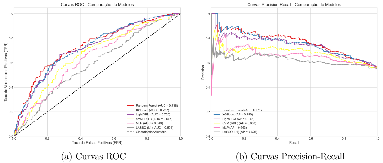
Figura 5.3: Curvas de avaliação de desempenho. (a) As curvas ROC mostram que os modelos de árvore dominam. (b) As curvas Precision-Recall confirmam essa tendência.
