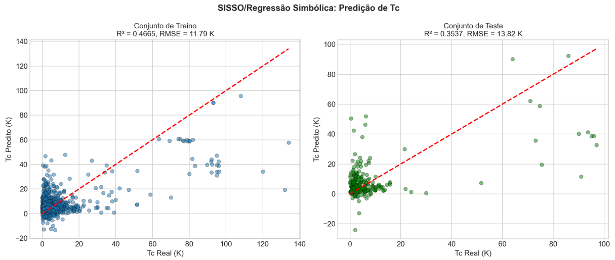
Figura 4.10: Predição de T_c pelo modelo SISSO. A dispersão dos pontos indica a complexidade do problema, mas a tendência geral é capturada.
