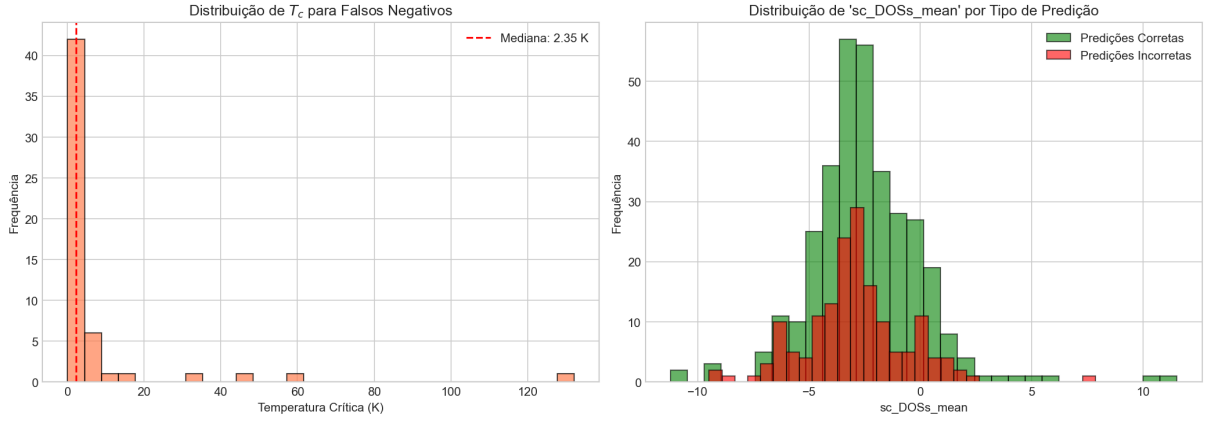
Figura 4.7: Análise de erro do modelo Random Forest. À esquerda, a distribuição de T_c para os Falsos Negativos. À direita, a distribuição da feature sc_DOSs_mean para predições corretas e incorretas.
