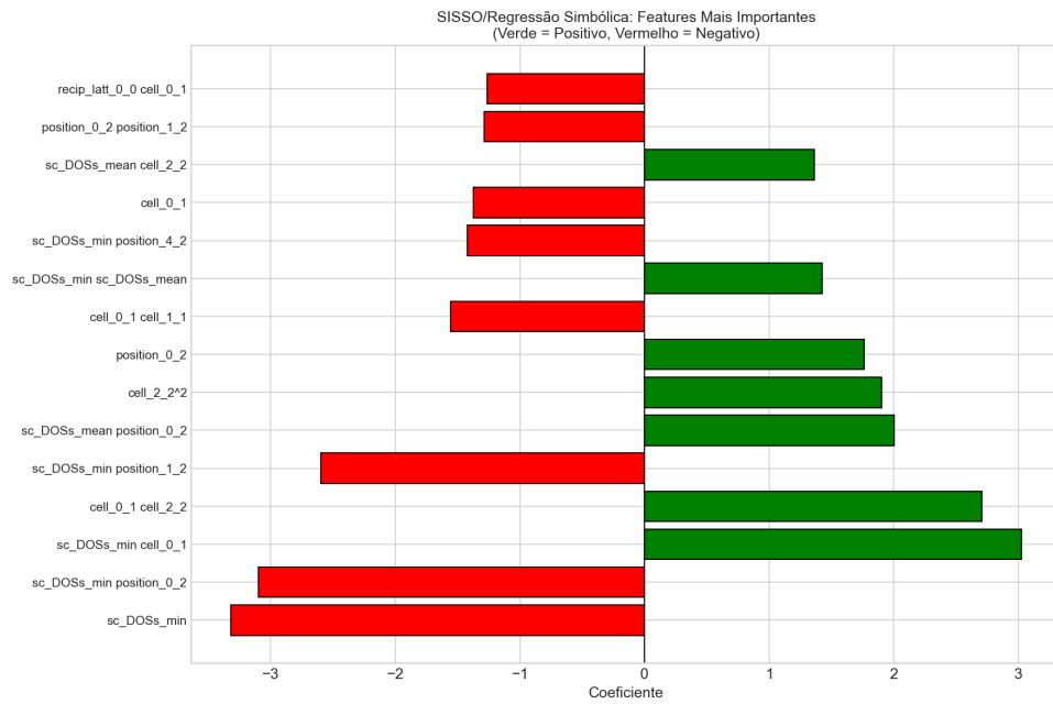
Figura 4.11: Coeficientes da equação descoberta pelo SISSO. A dominância de termos envolvendo a densidade de estados ( sc_DOSs_min ) é evidente.
