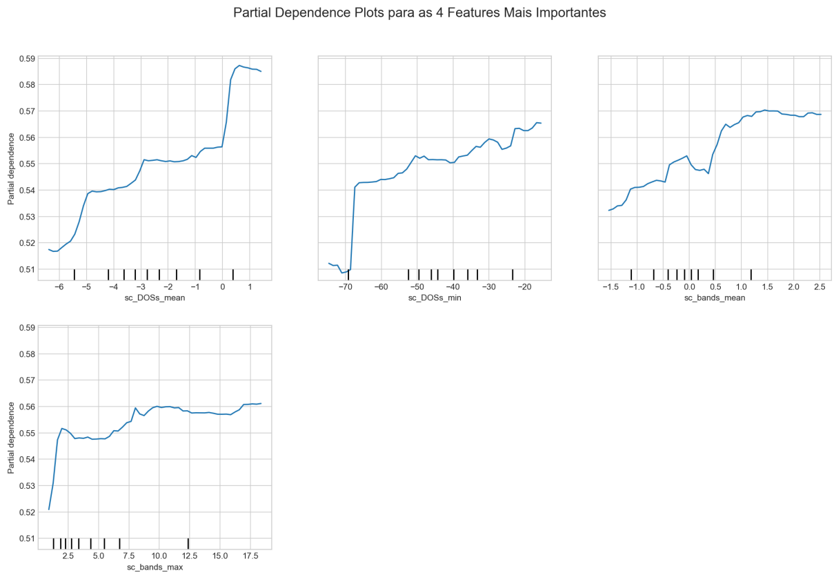
Figura 4.6: Partial Dependence Plots para as 4 features mais importantes do modelo Random Forest.
