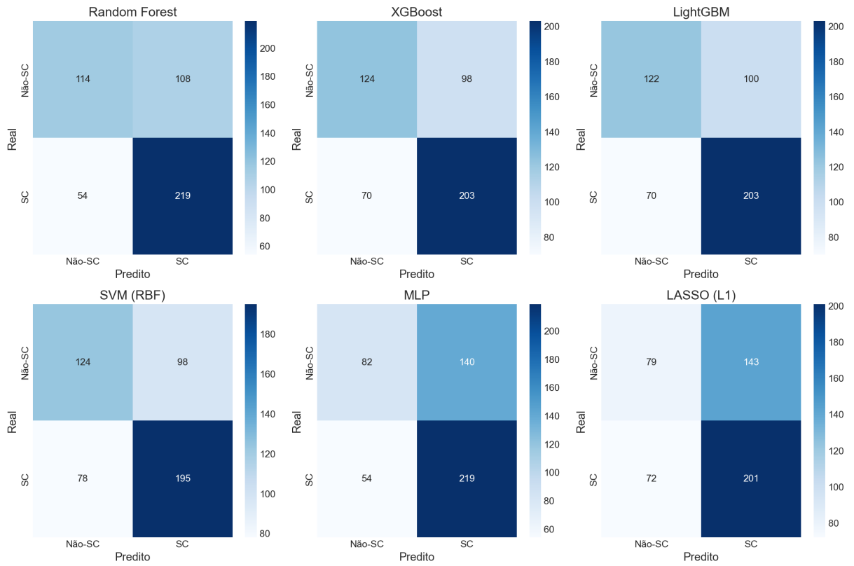
Figura 4.4: Matrizes de confusão para os seis modelos de aprendizado de máquina avaliados. Os valores representam o número de amostras em cada categoria.
