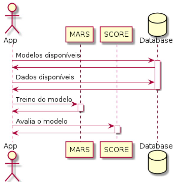
Figura 8 – Diagrama de Sequência - MARS
