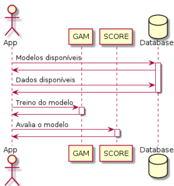
Figura 7 – Diagrama de Sequência - GAM
