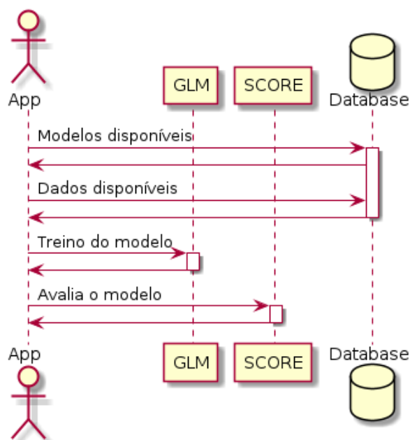
Figura 6 – Diagrama de Sequência - GLM
