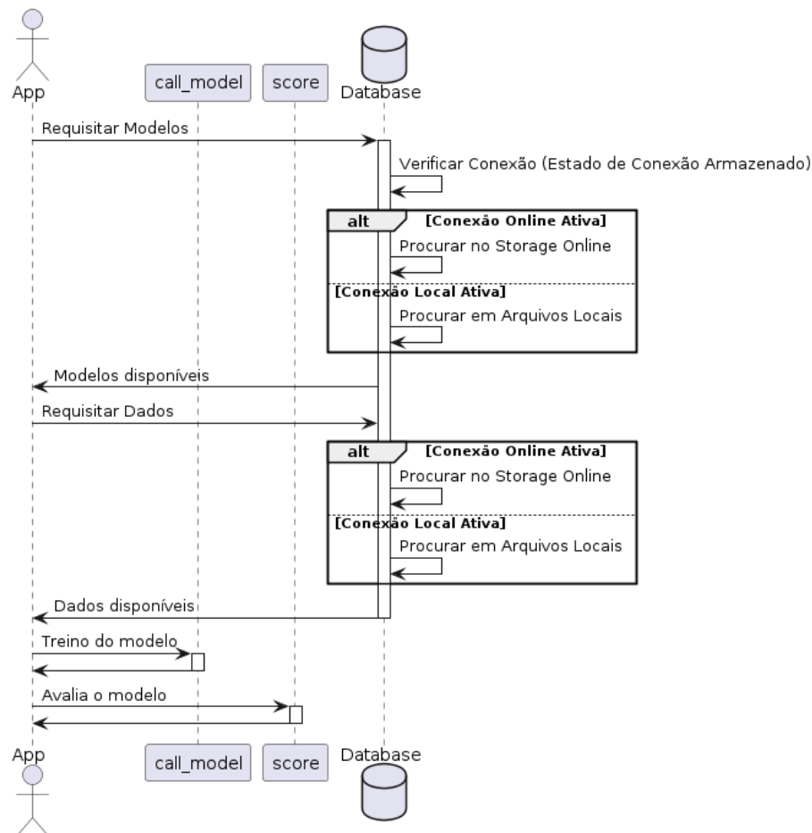
Figura 5 – Diagrama de Sequência - MODELO
