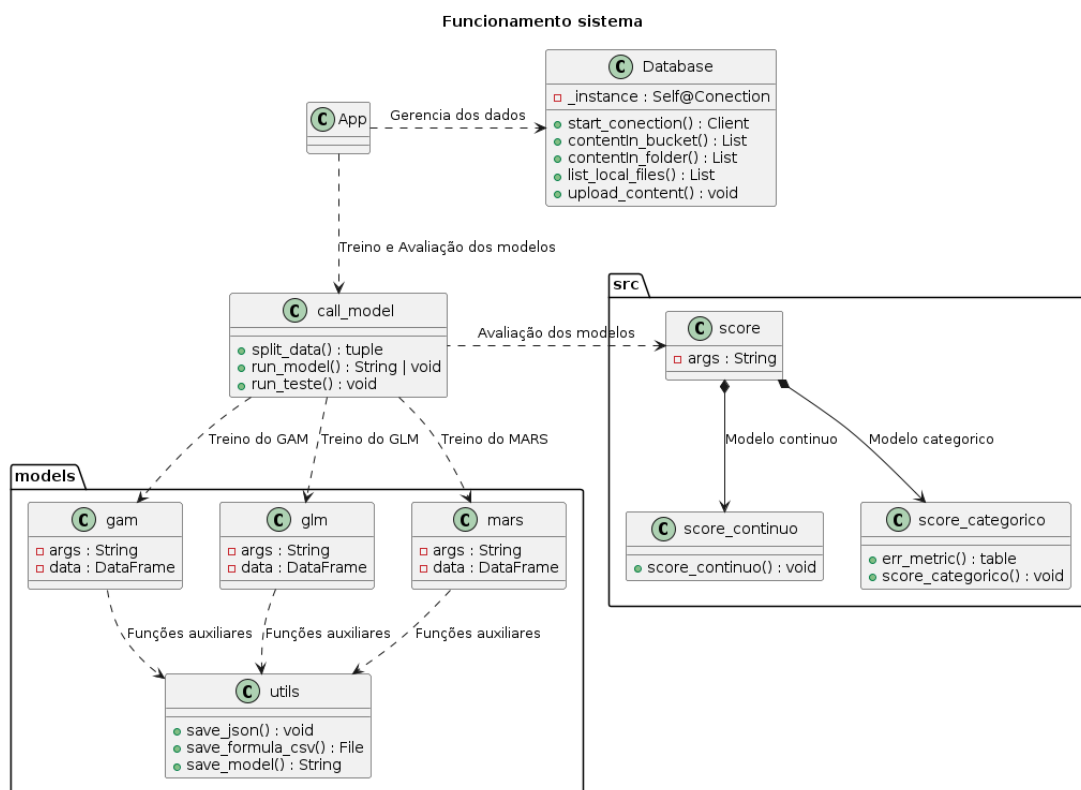
Figura 4 – Arquitetura do sistema
