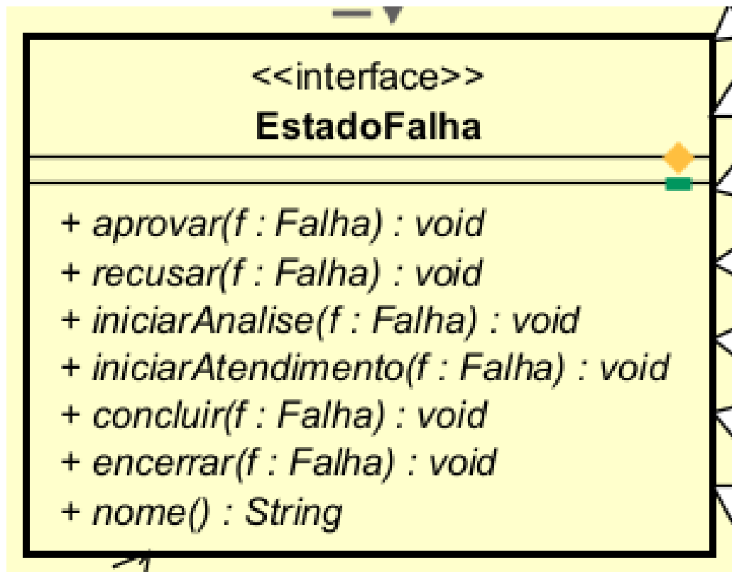
Figura 1: Diagrama de Classes - Padrão State
