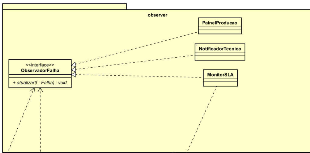
Figura 3: Diagrama de Classes - Padrão Observer
