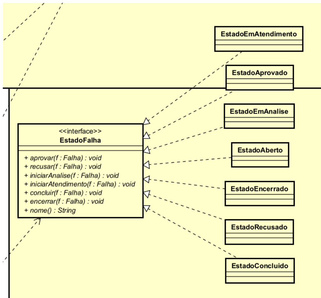
Figura 1: Diagrama de Classes - Padrão State
