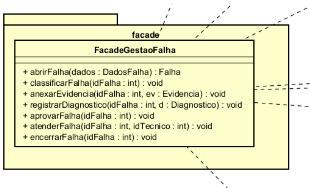
Figura 5: Diagrama de Classes - Padrão Facade
