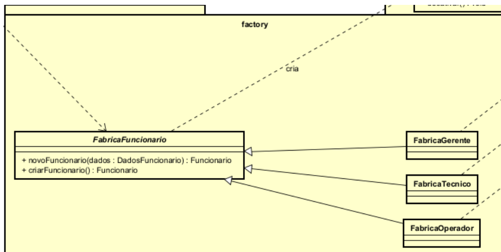
Figura 4: Diagrama de Classes - Padrão Factory Method
