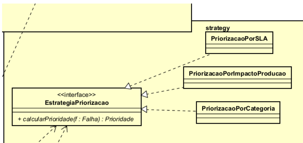
Figura 2: Diagrama de Classes - Padrão Strategy
