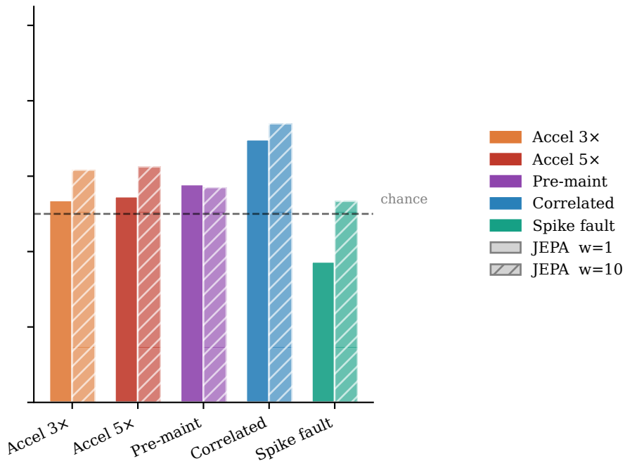
k-NN detector
