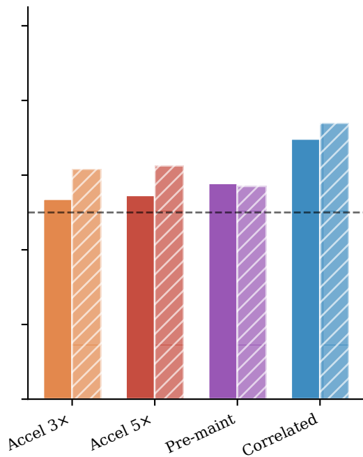
k-NN detector
