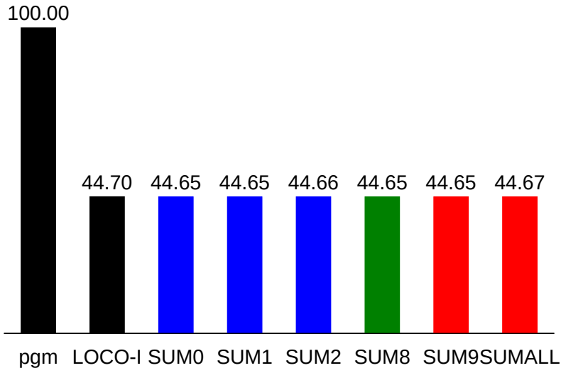
kodim23
