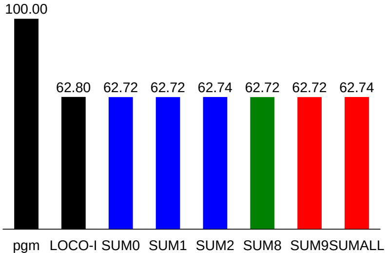
kodim14
