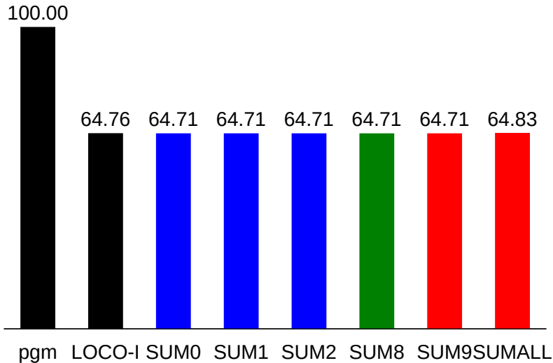
kodim18
