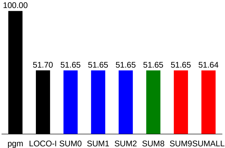
kodim16
