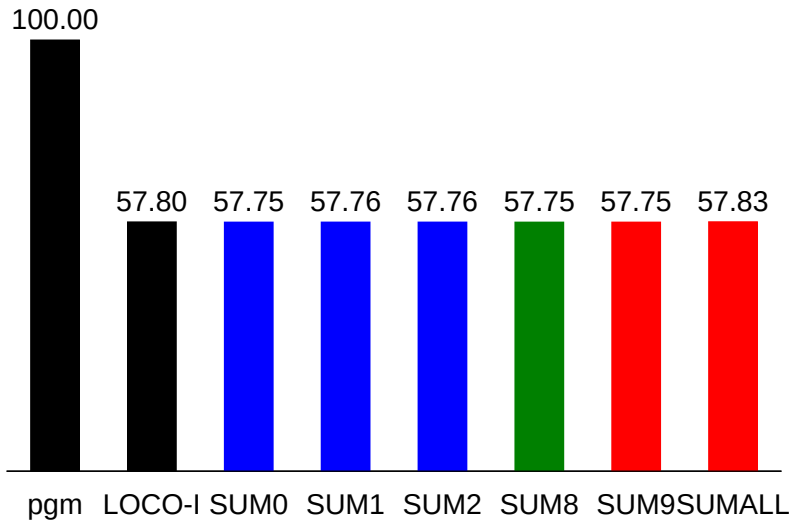
kodim22
