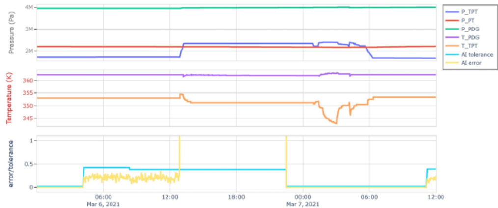
Figura 7.4: Exemplo de detecção em dados reais. Nos dois painéis superiores, as pressões e as temperaturas medidas por PDG e TPT; no inferior, o escore de anomalia com a linha de tolerância da Equação (7.1). A ultrapassagem do limiar precede em várias horas o desvio que seria visível a olho nu nos sinais brutos. Adaptado de Aranha et al. (2024a).
