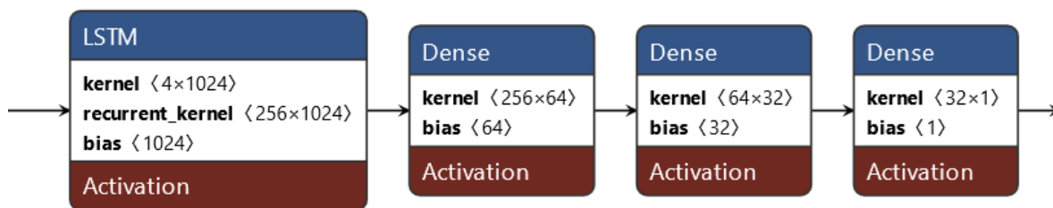
Figura 11.1: Classificador binário aplicado ao segmento identificado, com as dimensões efetivas de cada tensor de parâmetros: uma camada recorrente seguida de camadas densas decrescentes até uma única saída escalar. A figura mostra a variante com LSTM de 256 unidades; o número de unidades recorrentes é ajustado por classe. Adaptado de Lopes et al. (2026a).
