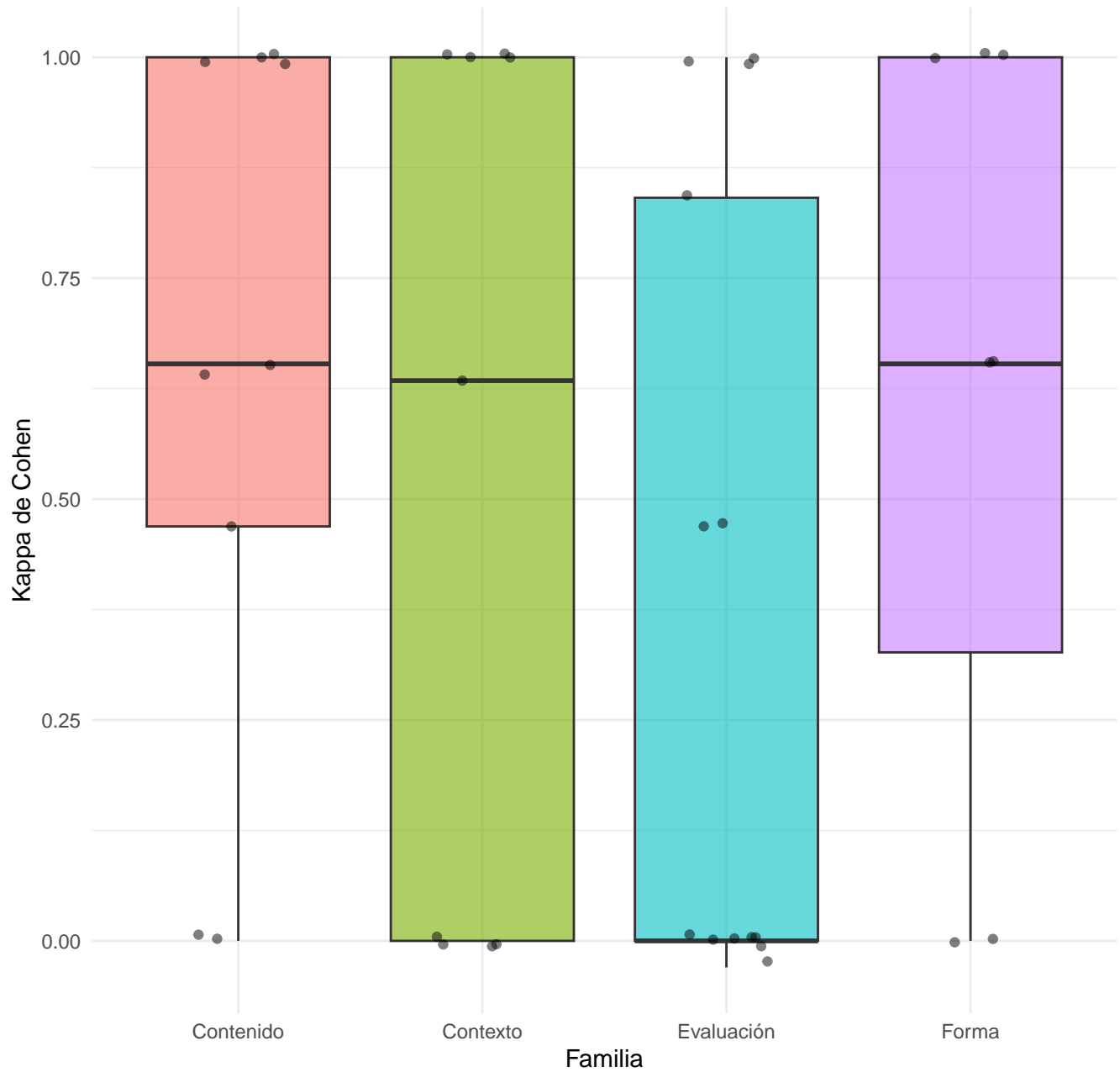
Distribución de Kappa por Familia de Códigos
