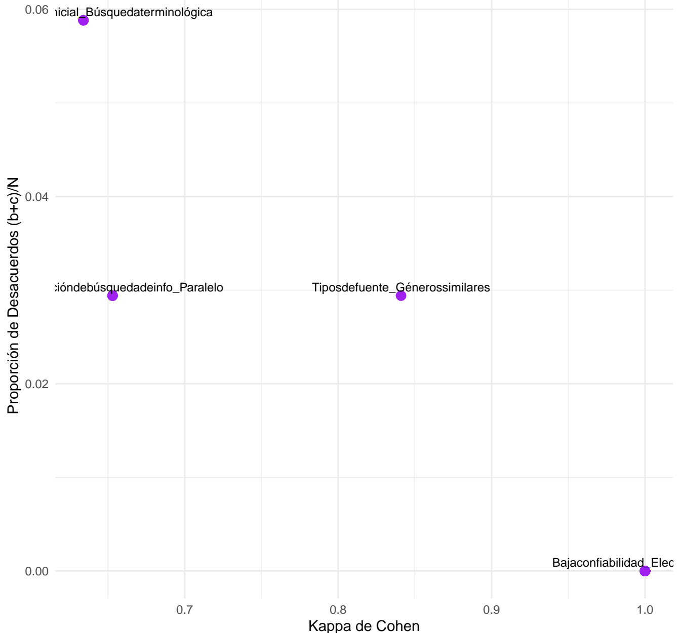
Kappa vs Proporción de Desacuerdos (Códigos Clave)
