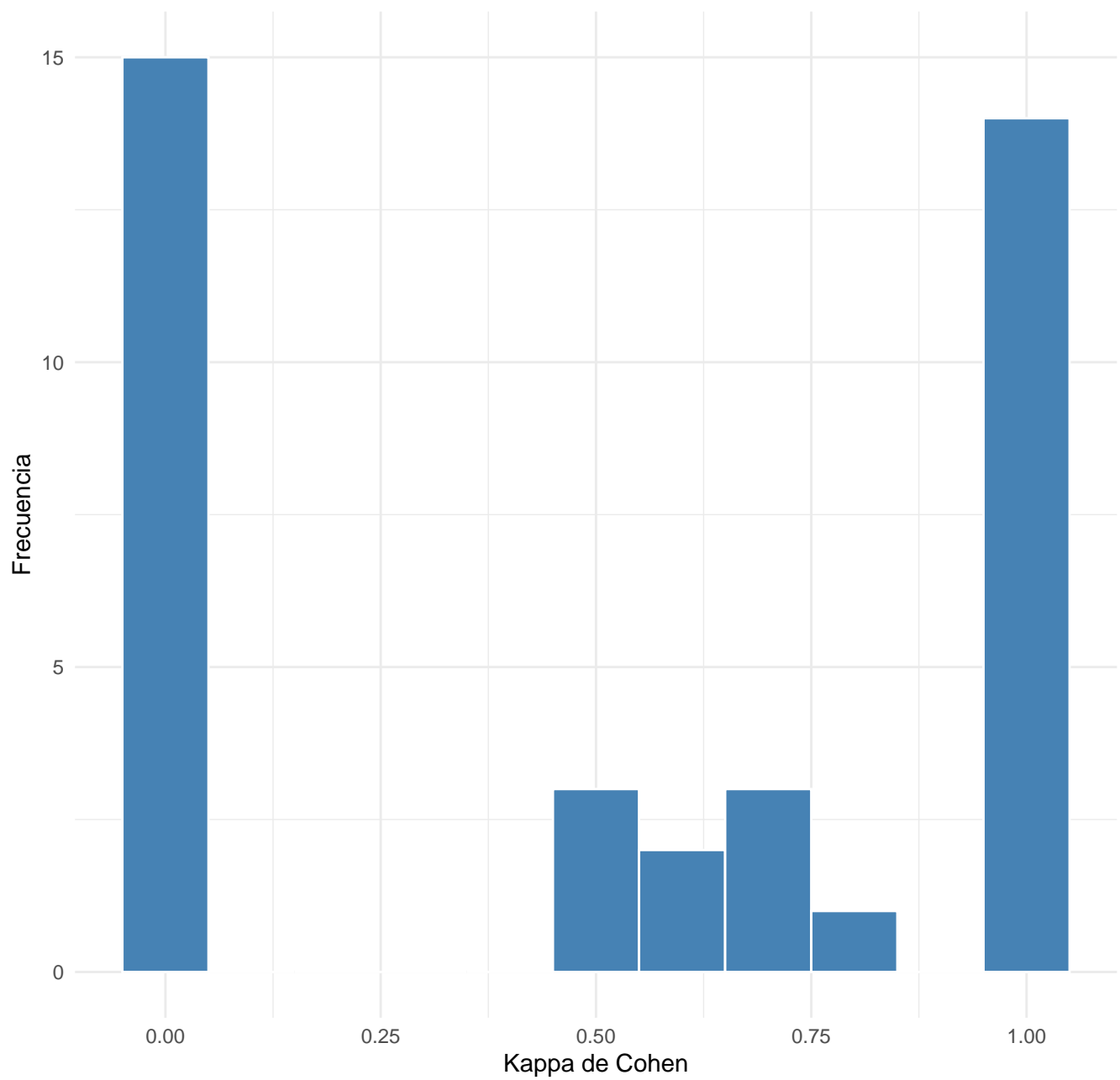
Distribución de Kappa por Código
