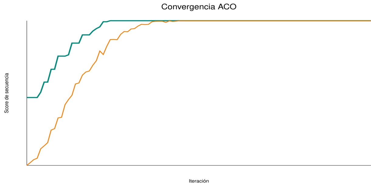
Figura C.2. Evolución del mejor puntaje y del promedio de la población. El algoritmo parte con un mejor valor de 0,666753, supera el 99 % del resultado final en la iteración 20 y alcanza su mejor solución, 0,730704, en la iteración 24. La estabilización posterior indica convergencia del proceso de búsqueda.
