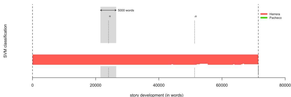
Figura 4. Resultado de aplicar Rolling Classify mediante la técnica Rolling SVM a la totalidad de los poemas de Versos .
