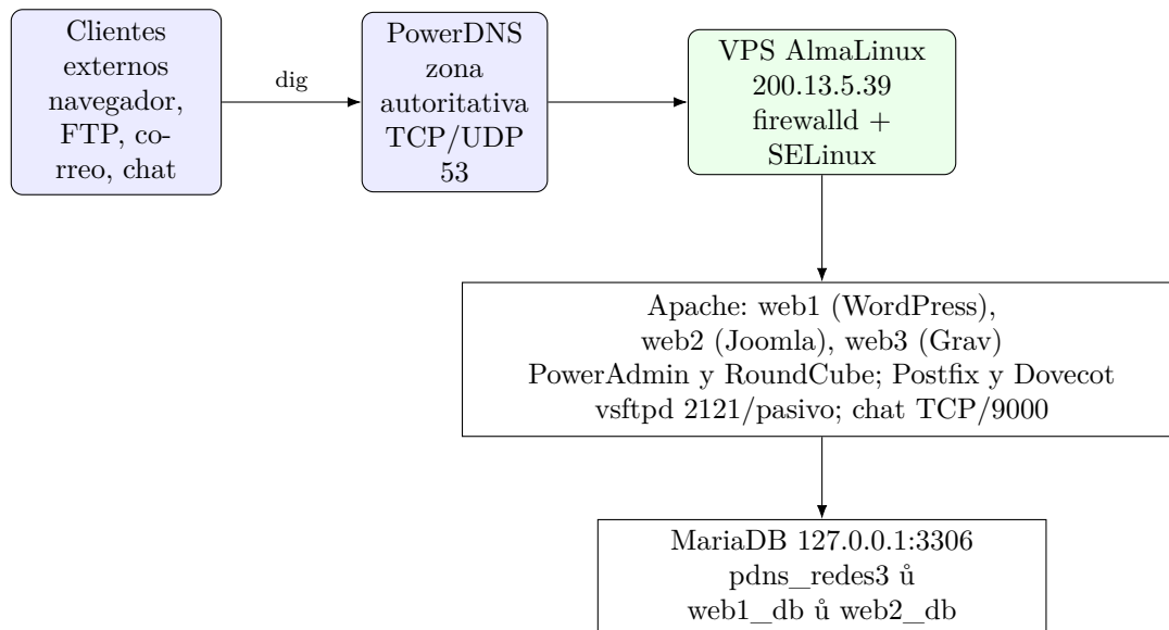
Figura 3: Arquitectura general del VPS. Las flechas representan dependencias entre cliente, aplicaciones y persistencia; no son capturas de funcionamiento. Grav guarda páginas en archivos y no usa MariaDB.
