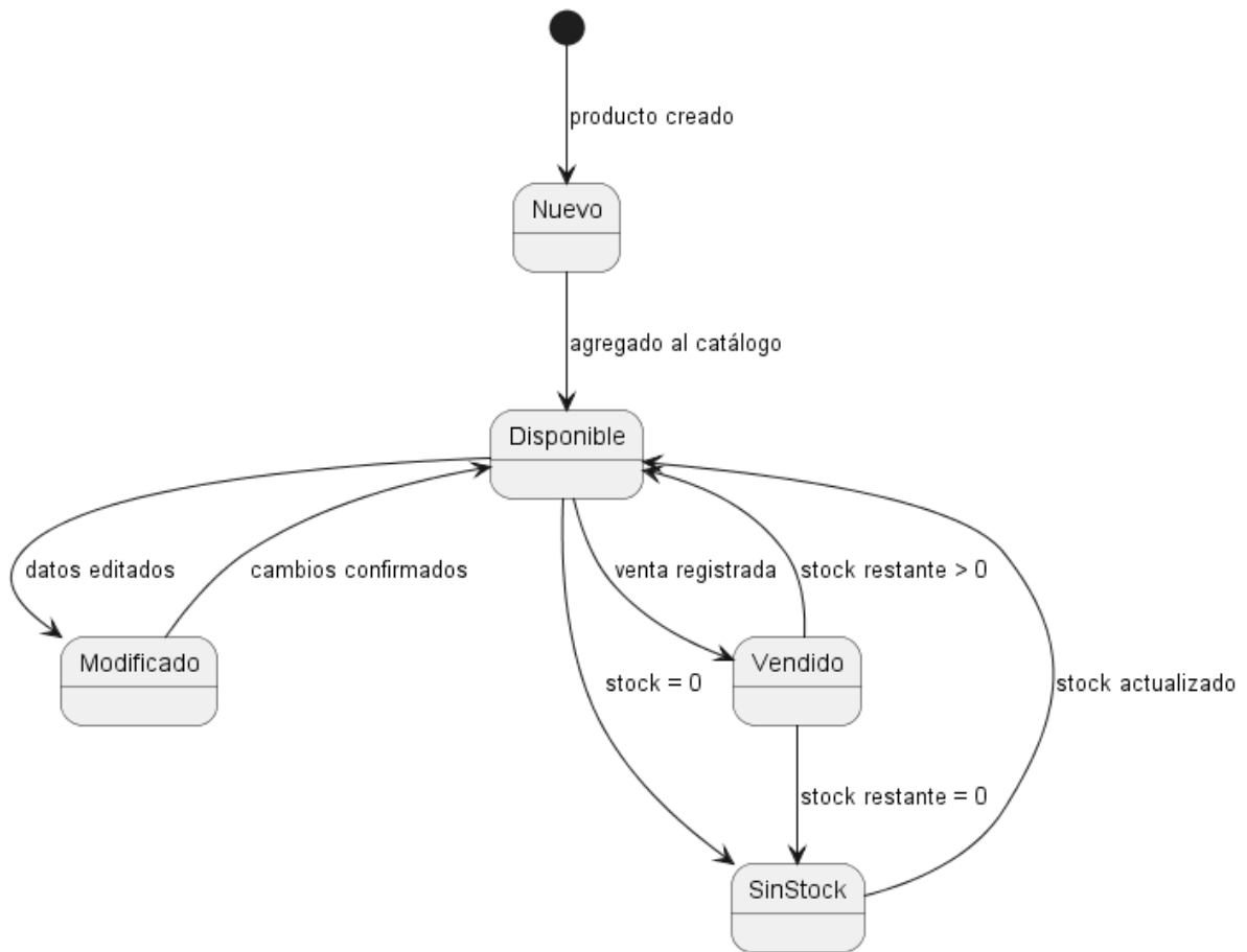
Diagrama de Estados - Producto
