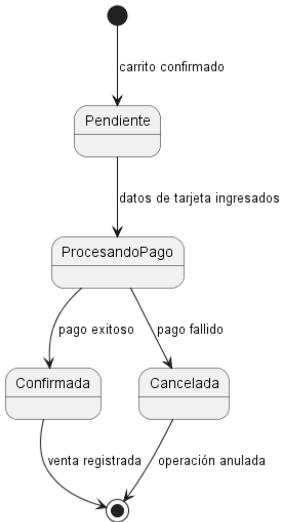
Diagrama de Estados - Venta
