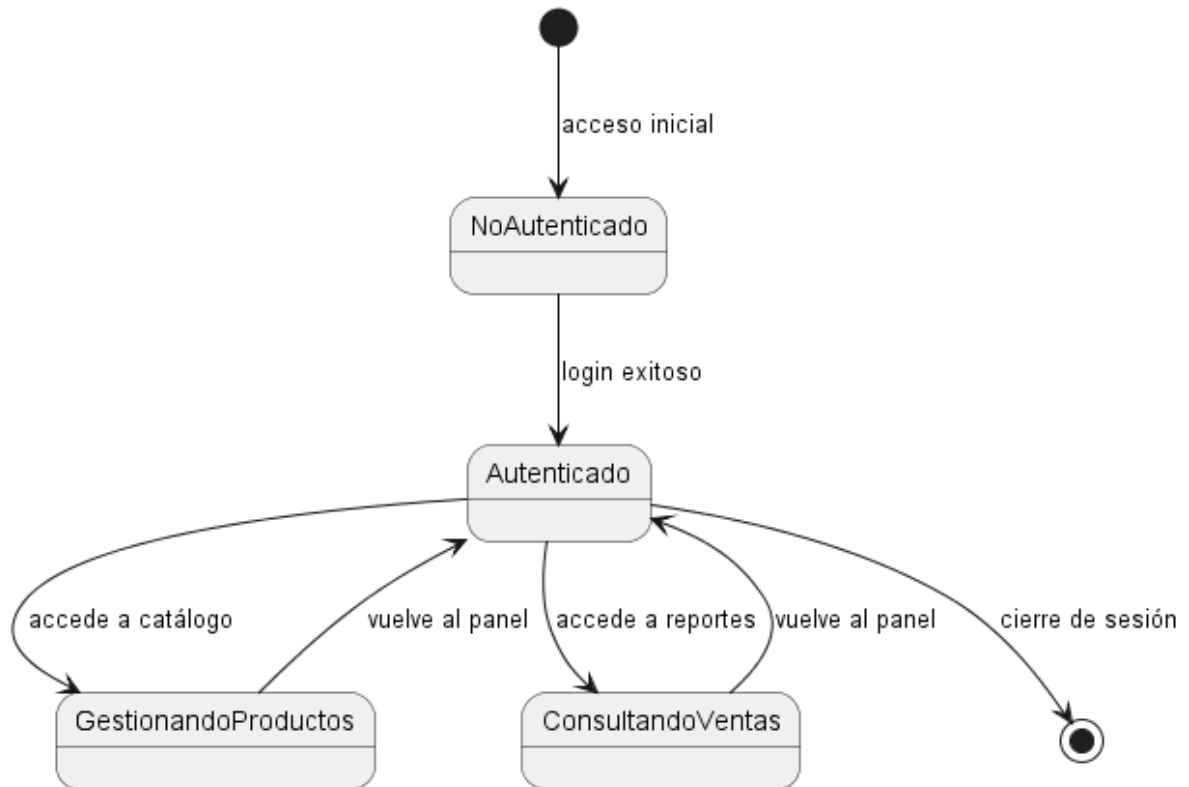
Diagrama de Estados - Administrador
