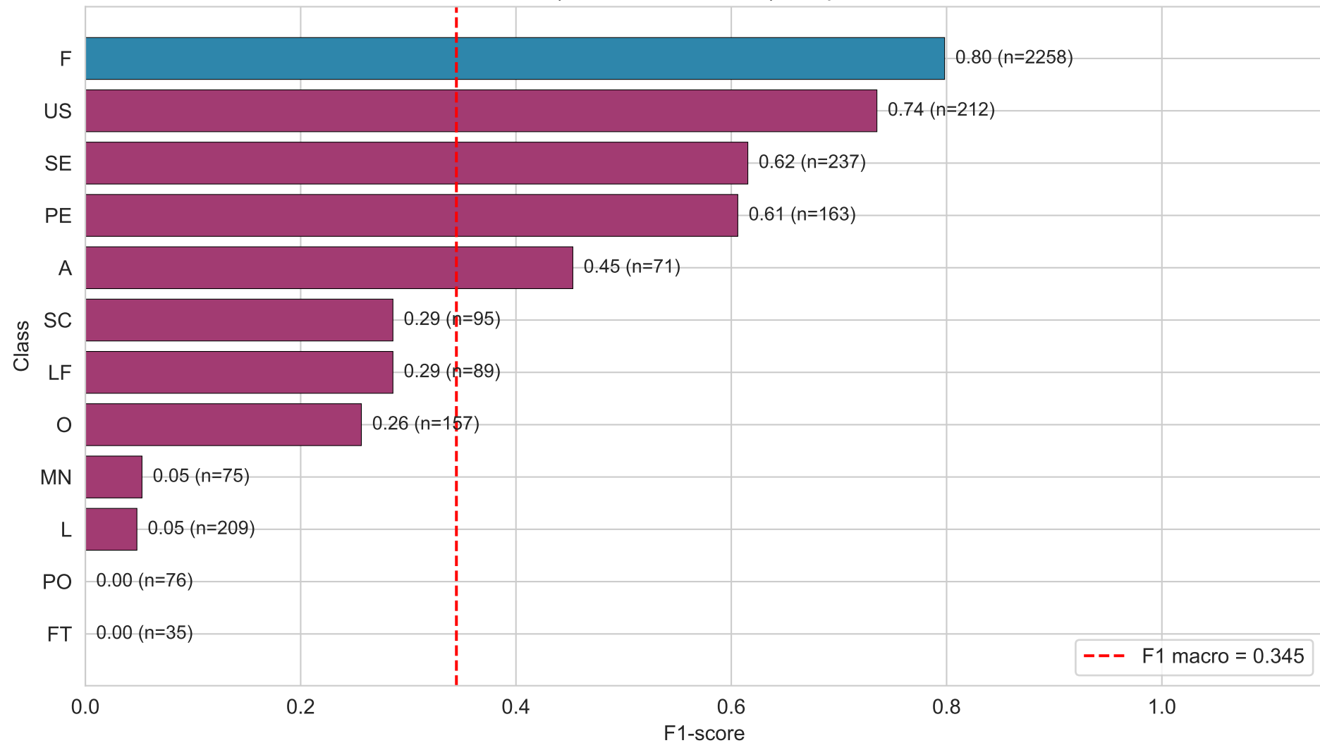
BERT (bert-base-uncased): F1 per class
