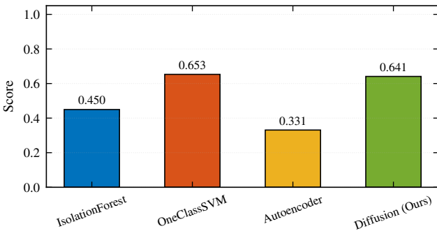
Precision
