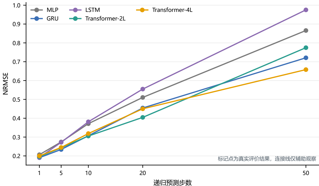
M1000: 多步递归预测误差累积
