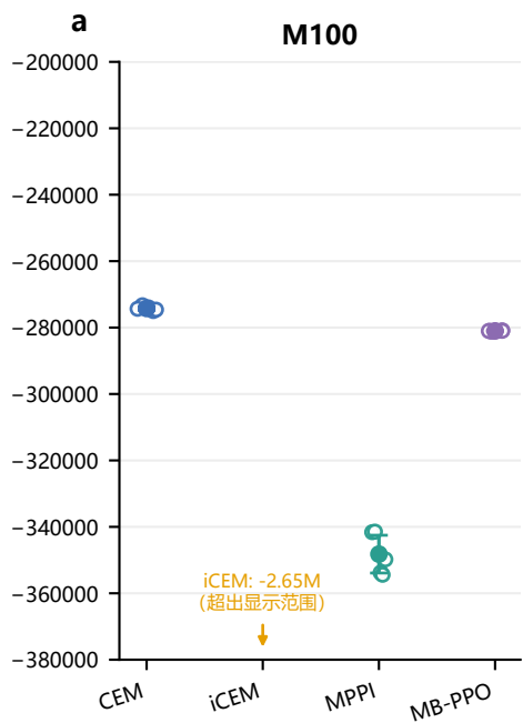
1000步累计奖励 (越高越好)
