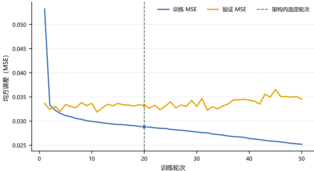
M1000 Transformer-2L: 正式50轮训练历史
