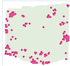
GSE274657
