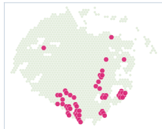
GSE211956
