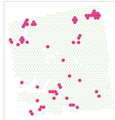
GSE288483
