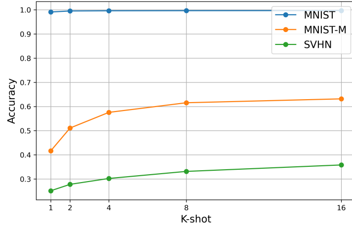
Figura 4: Accuracy sobre el conjunto de test de MNIST con k = 1, 2, 4, 8, 16 .
