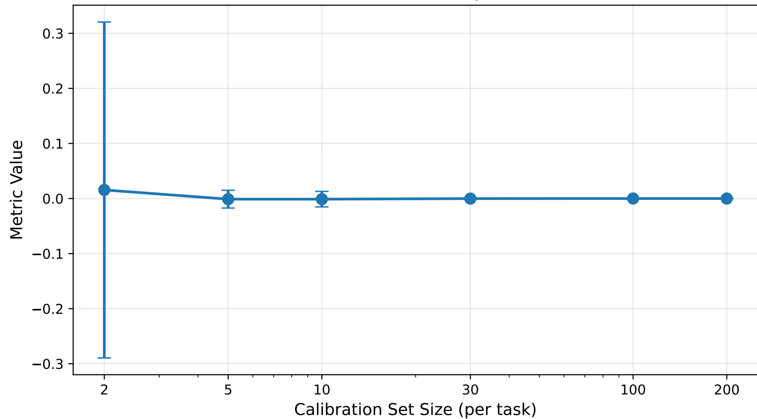
encoder_gradient_dot_product Mean \pm Std across pairs
