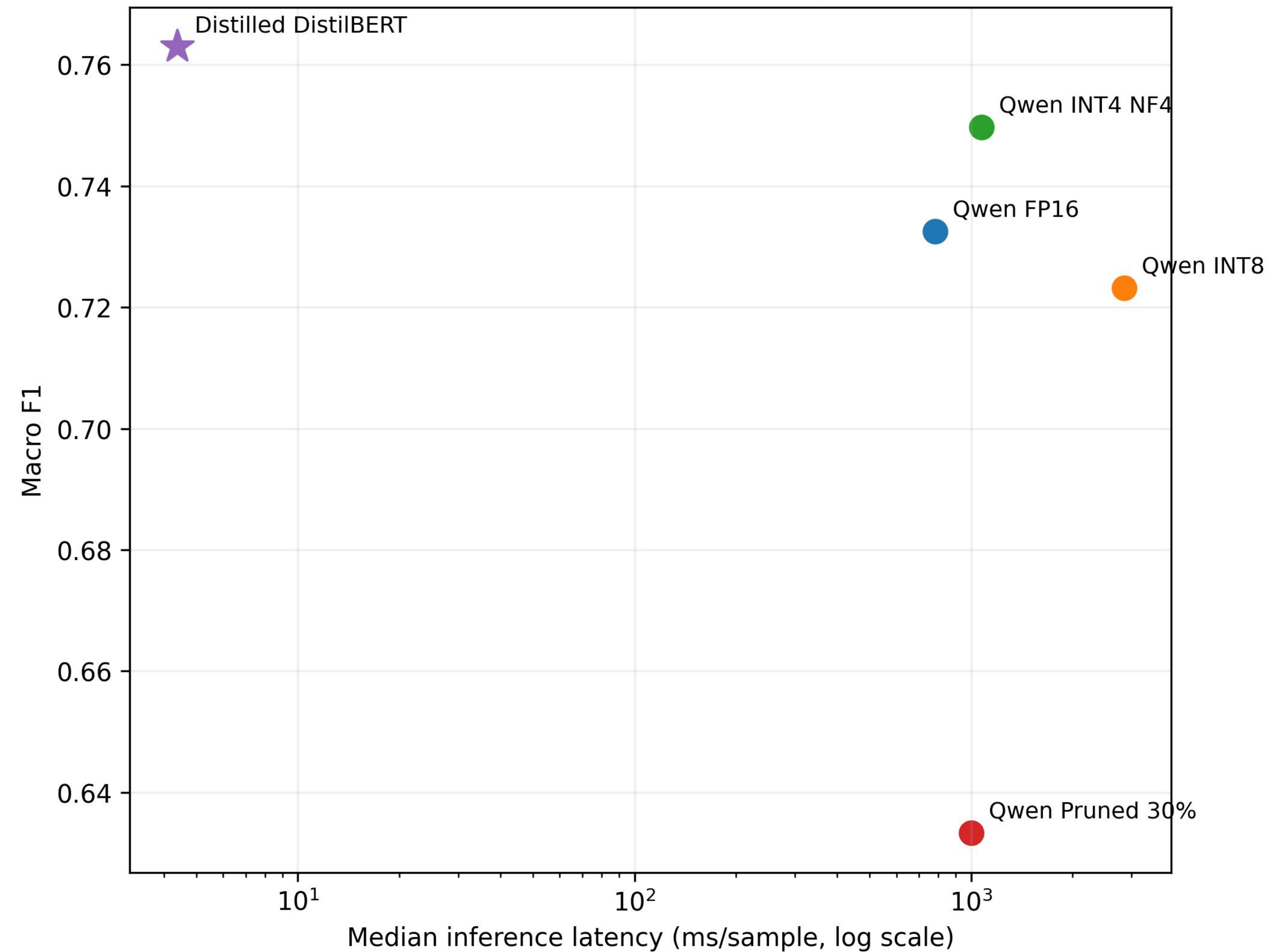
B. Macro F1 vs. Latency
