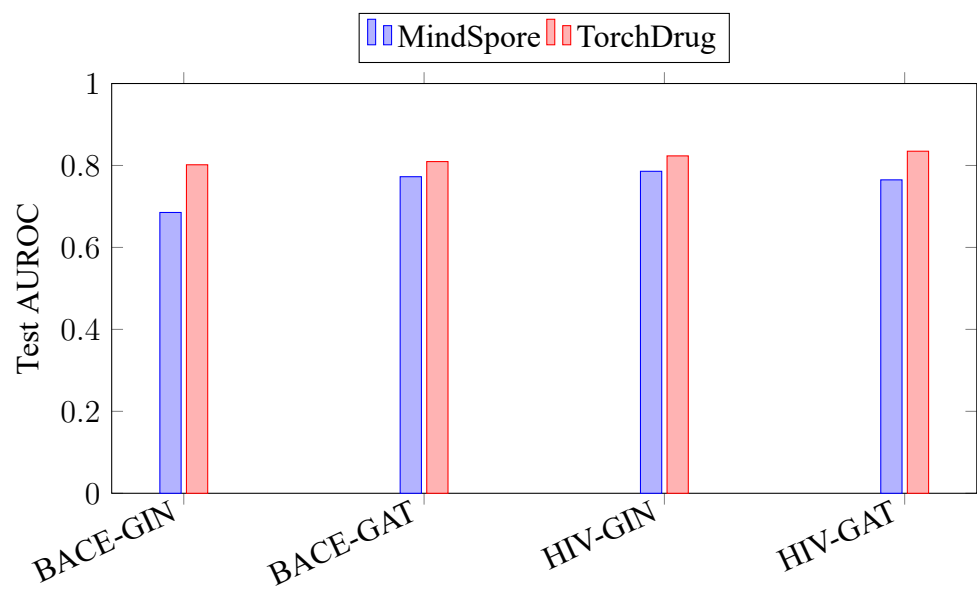
图 4: MindSpore 与 TorchDrug 测试集 AUROC 对比
