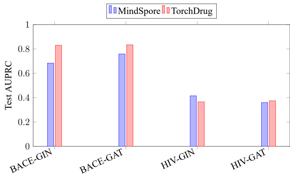
图 5: MindSpore 与 TorchDrug 测试集 AUPRC 对比
