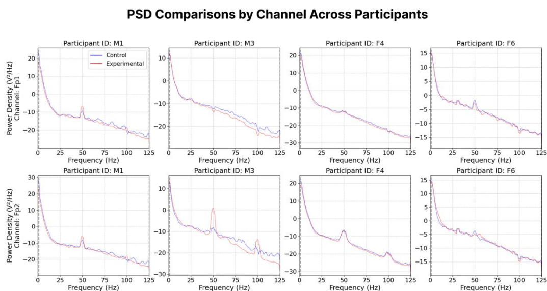
图 8.7 四名参与者在控制组（蓝线）与实验组（红线）条件下，FP1 和 FP2 通道的功率谱密度（PSD）对比。
