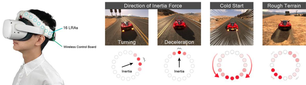
图 2.8 DrivingVibe [134] 系统利用头戴式多点震动阵列模拟连续的空间物理隐喻
