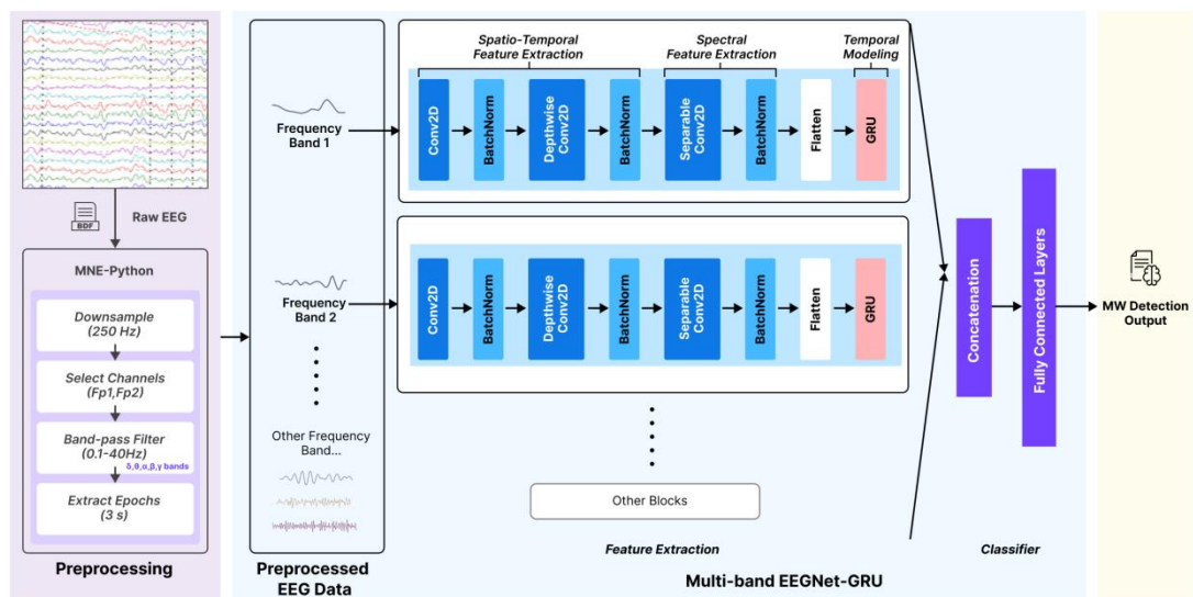
图 6.1 EEGNet-GRU 的心智游移检测算法整体架构
