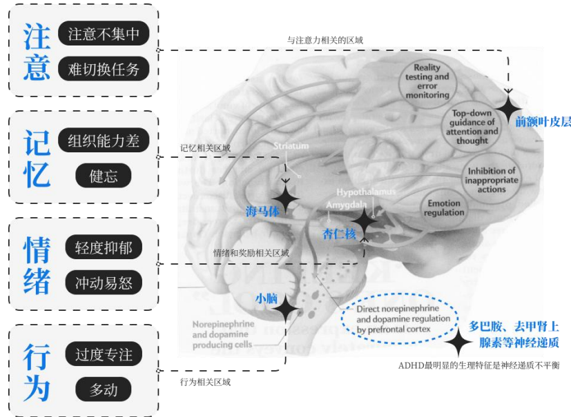
图 2.1 ADHD 的核心症状（注意、记忆、情绪、行为）与大脑关键区域（前额叶、海马体、杏仁核、小脑）及神经递质异常的生理机制映射图
