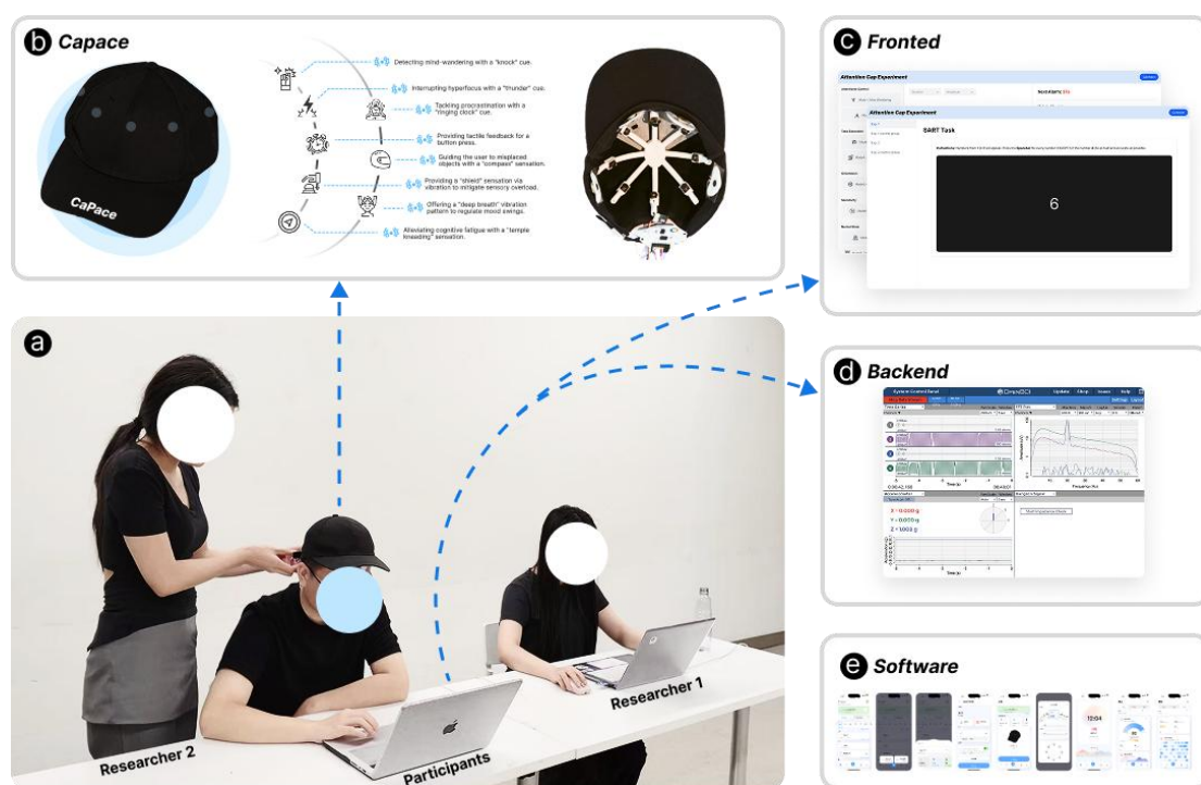
图 8.1 实验设置: (a) 用户实验环境; (b) Capace 帽子; (c) 模拟任务实验页面; (d) 脑电数据记录后端; (e) 真实场景任务使用软硬件
