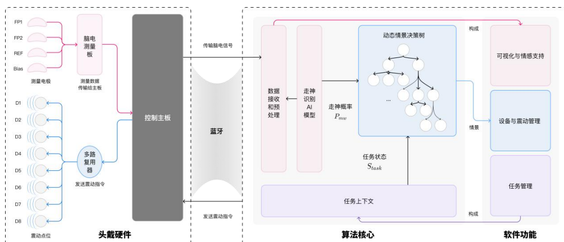
图 4.6 Capace 软硬件架构
