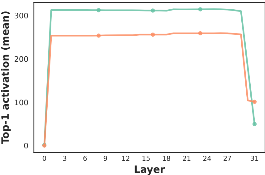
Mistral-7B
