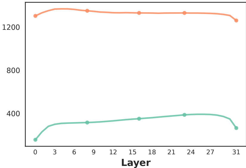
OPT-6.7B
