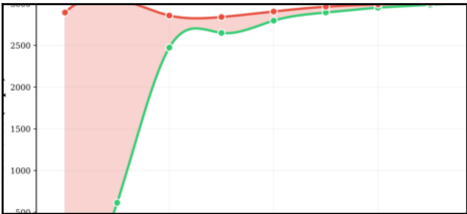
GPT-2
