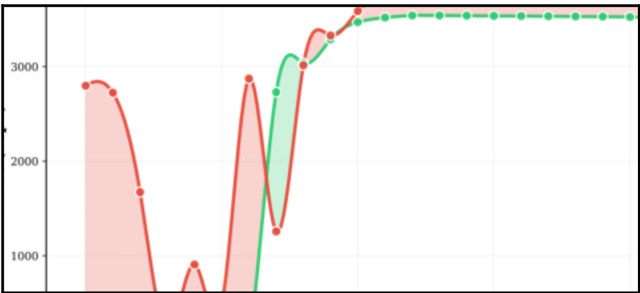
BLOOM-7B1
