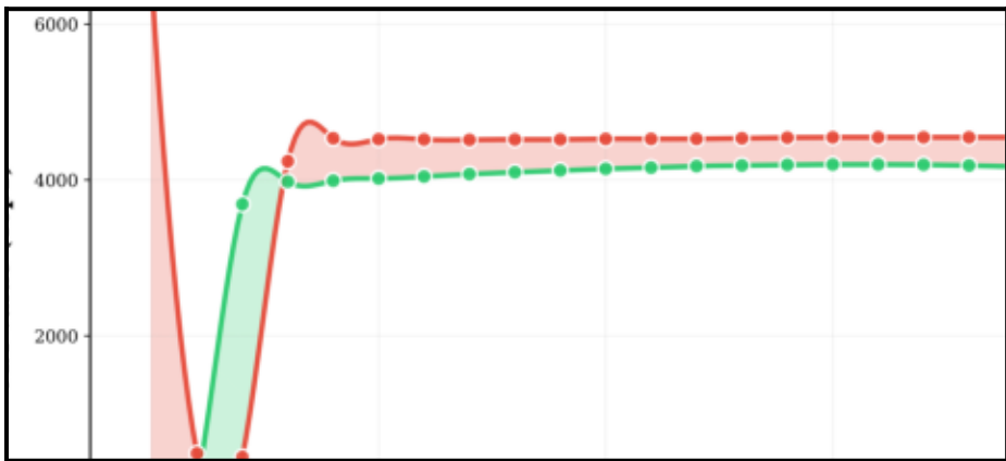
GPT-J-6B
