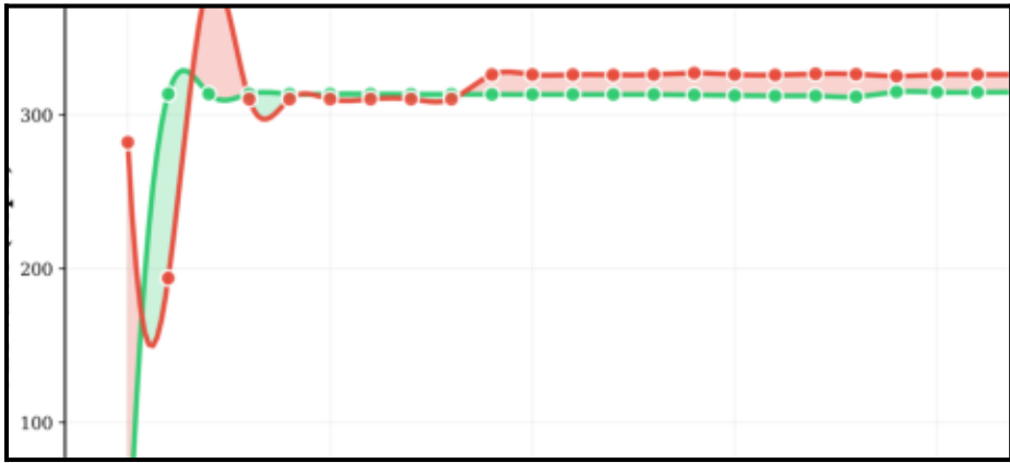
Mistral-7B
