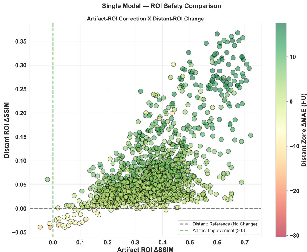
Fig.5.16 Relação por imagem entre a melhoria de SSIM \setminus PSNR na Zona de Artefacto e a alteração de SSIM \setminus PSNR na Zona Limpa para o Single Model, seed 2024. A cor codifica a redução de MAE na Zona Limpa.
