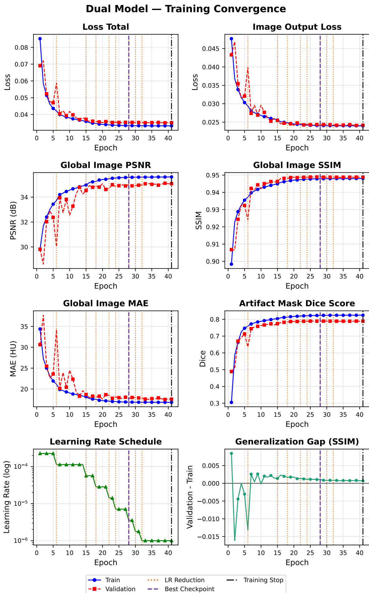
Fig.5.9 Curvas de convergência para seed_1337/training_001_dualhead . Linhas verticais laranjas pontilhadas: reduções da taxa de aprendizagem; linha roxa tracejada: época do melhor checkpoint segundo o SSIM de validação; linha preta traço-ponto: interrupção do treino. O painel de generalization gap representa validação menos treino para o SSIM e permite identificar divergência persistente compatível com sobreajuste.
