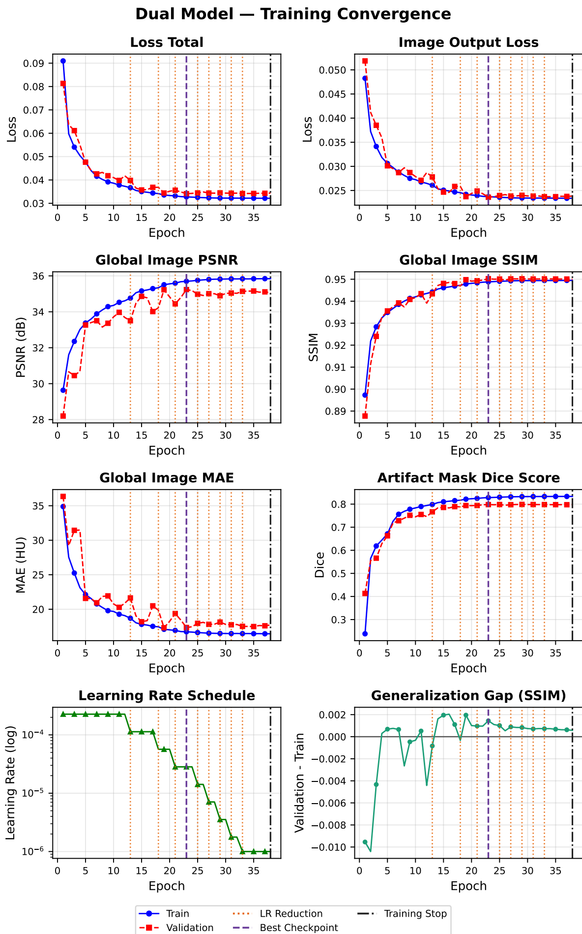
Fig.5.11 Curvas de convergência para seed_2024/training_001_dualhead . Linhas verticais laranjas pontilhadas: reduções da taxa de aprendizagem; linha roxa tracejada: época do melhor checkpoint segundo o SSIM de validação; linha preta traço-ponto: interrupção do treino. O painel de generalization gap representa validação menos treino para o SSIM e permite identificar divergência persistente compatível com sobreajuste.
