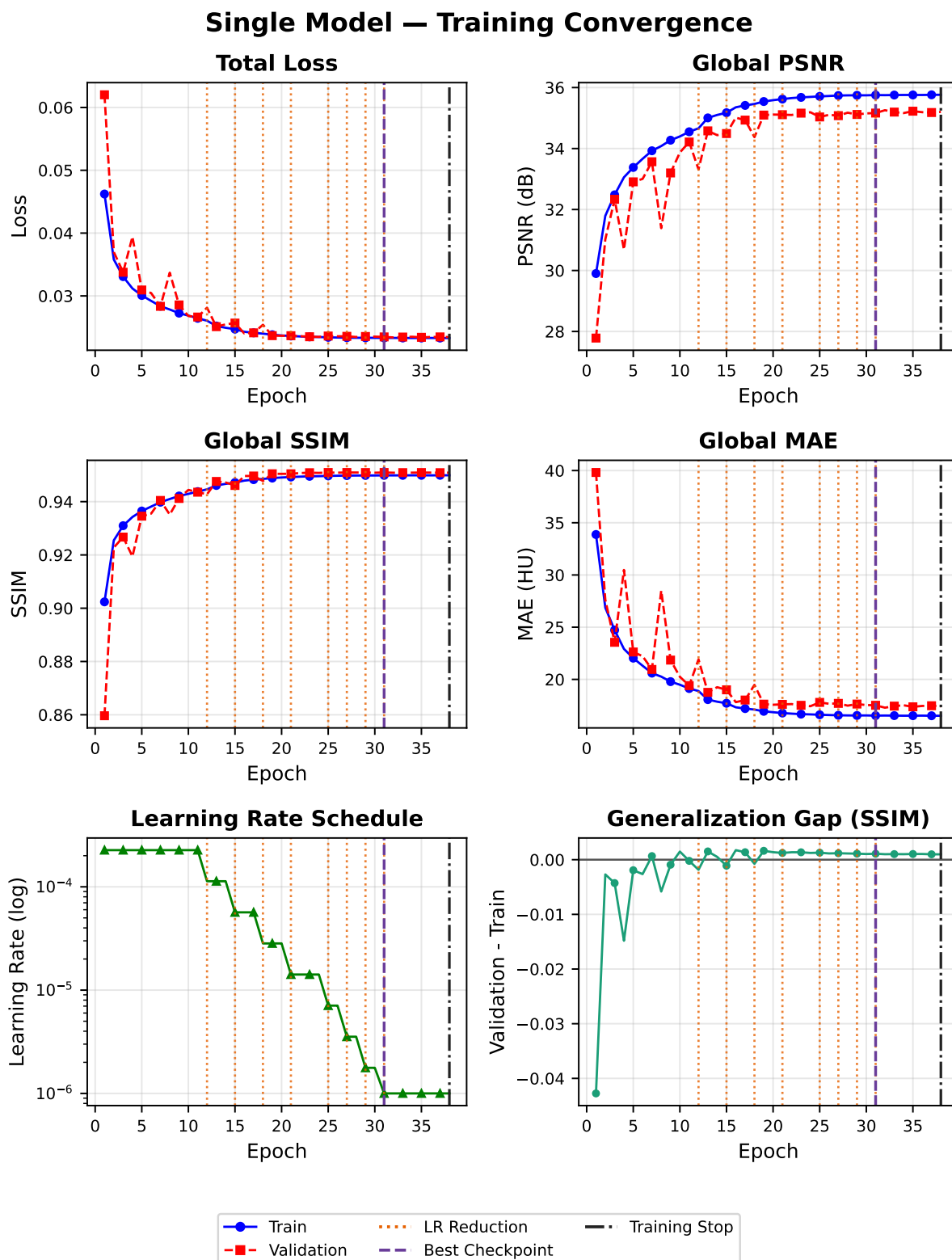
Fig.5.12 Curvas de convergência para seed_42/training_001_singlehead . Linhas verticais laranja pontilhadas: reduções da taxa de aprendizagem; linha roxa tracejada: época do melhor checkpoint segundo o SSIM de validação; linha preta traço-ponto: interrupção do treino. O painel de generalization gap representa validação menos treino para o SSIM e permite identificar divergência persistente compatível com sobreajuste.
