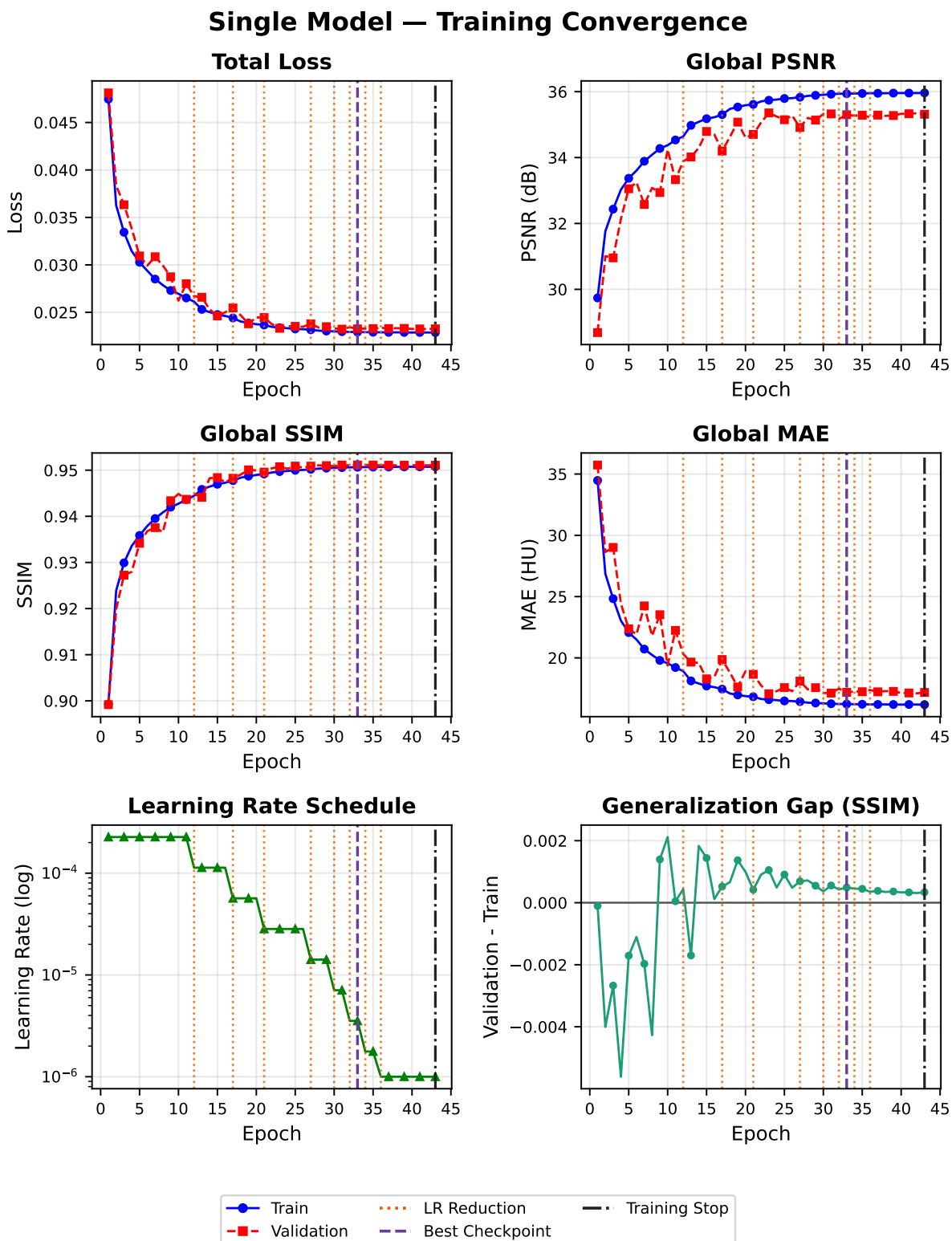
Fig.5.10 Curvas de convergência para seed_2024/training_001_singlehead . Linhas verticais laranja pontilhadas: reduções da taxa de aprendizagem; linha roxa tracejada: época do melhor checkpoint segundo o SSIM de validação; linha preta traço-ponto: interrupção do treino. O painel de generalization gap representa validação menos treino para o SSIM e permite identificar divergência persistente compatível com sobreajuste.
