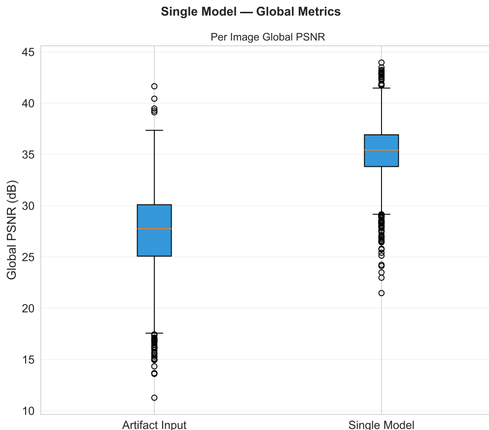
Fig.5.14 Distribuições por fatia do SSIM e do PSNR globais para o Single Model, seed 2024.
