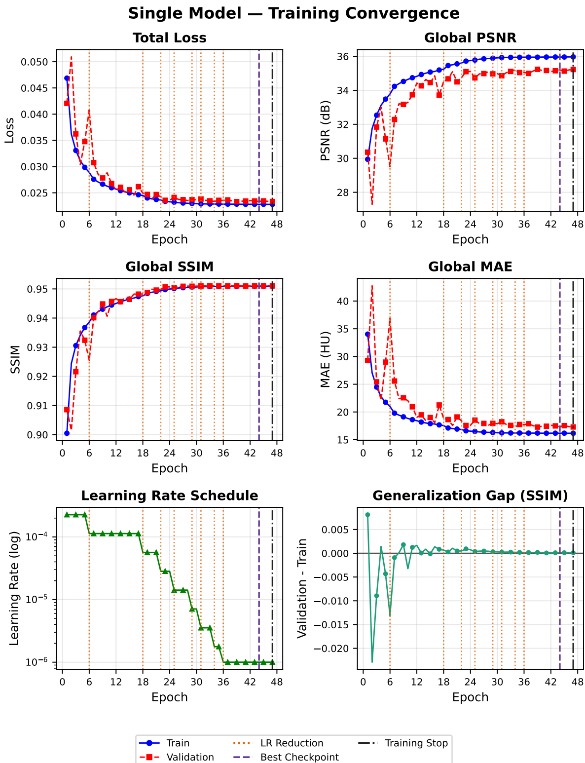
Fig.5.8 Curvas de convergência para seed_1337/training_008_singlehead . Linhas verticais laranjas pontilhadas: reduções da taxa de aprendizagem; linha roxa tracejada: época do melhor checkpoint segundo o SSIM de validação; linha preta traço-ponto: interrupção do treino. O painel de generalization gap representa validação menos treino para o SSIM e permite identificar divergência persistente compatível com sobreajuste.
