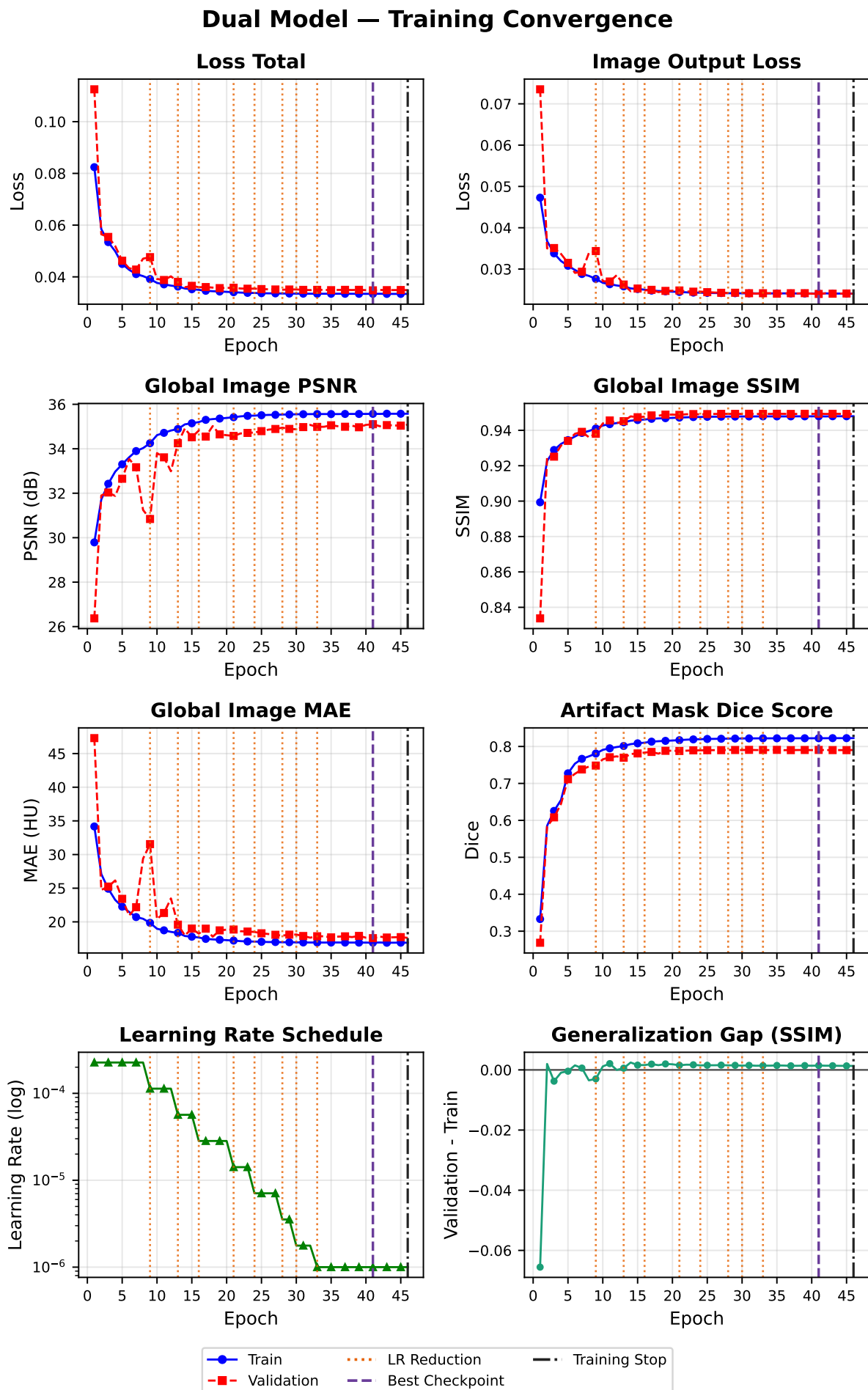
Fig.5.13 Curvas de convergência para seed_42/training_001_dualhead . Linhas verticais laranjas pontilhadas: reduções da taxa de aprendizagem; linha roxa tracejada: época do melhor checkpoint segundo o SSIM de validação; linha preta traço-ponto: interrupção do treino. O painel de generalization gap representa validação menos treino para o SSIM e permite identificar divergência persistente compatível com sobreajuste.
