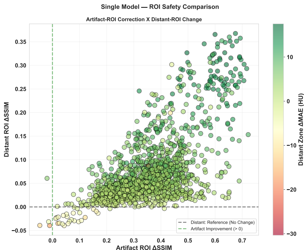
Fig.5.16 Relação por imagem entre a melhoria de SSIM \ PSNR na Zona de Artefacto e a alteração de SSIM \ PSNR na Zona Distante para o Single Model, seed 2024. A cor codifica a redução de MAE na Zona Distante.
