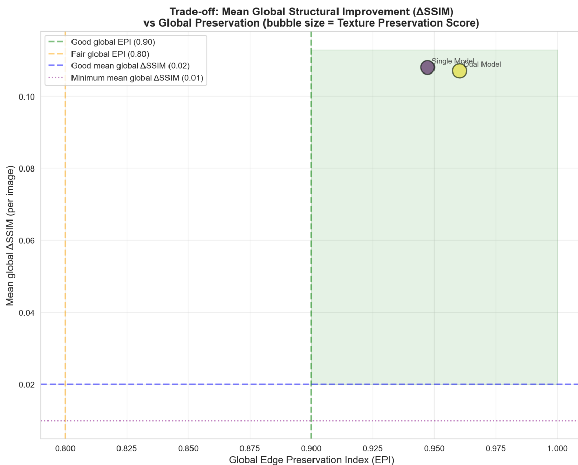
Fig.5.38 Comparacao entre modelos: comparison_scatter_tradeoff.png.
