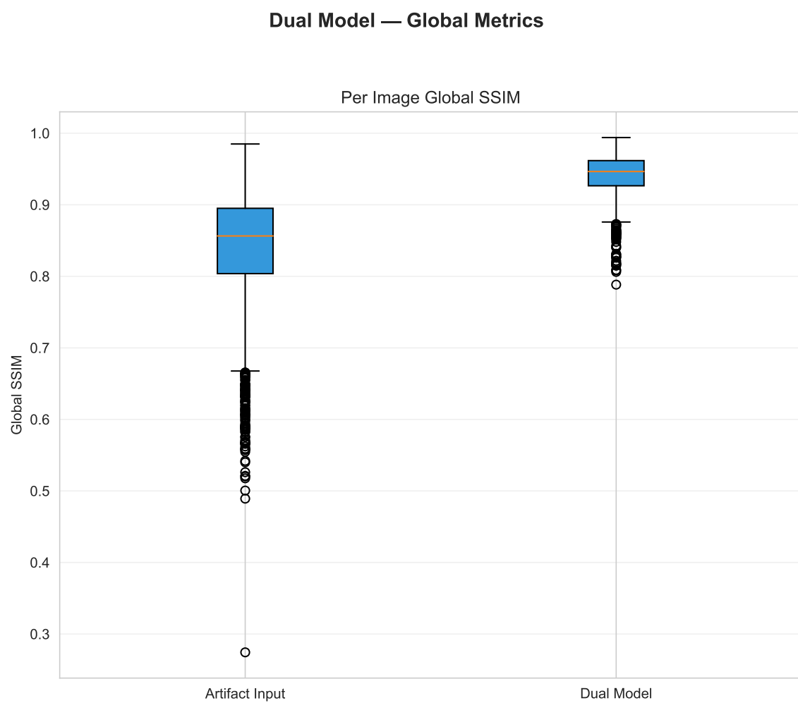
Fig.5.29 Distribuicao de metricas e analise de correlacao: boxplot_global_ssim_distribution.pdf.
