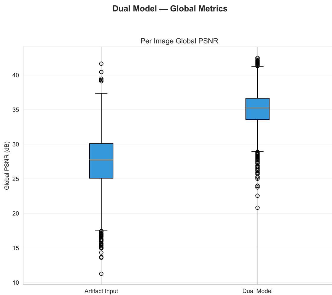
Fig.5.27 Distribuicao de metricas e analise de correlacao: boxplot_global_psnr_distribution.pdf .
