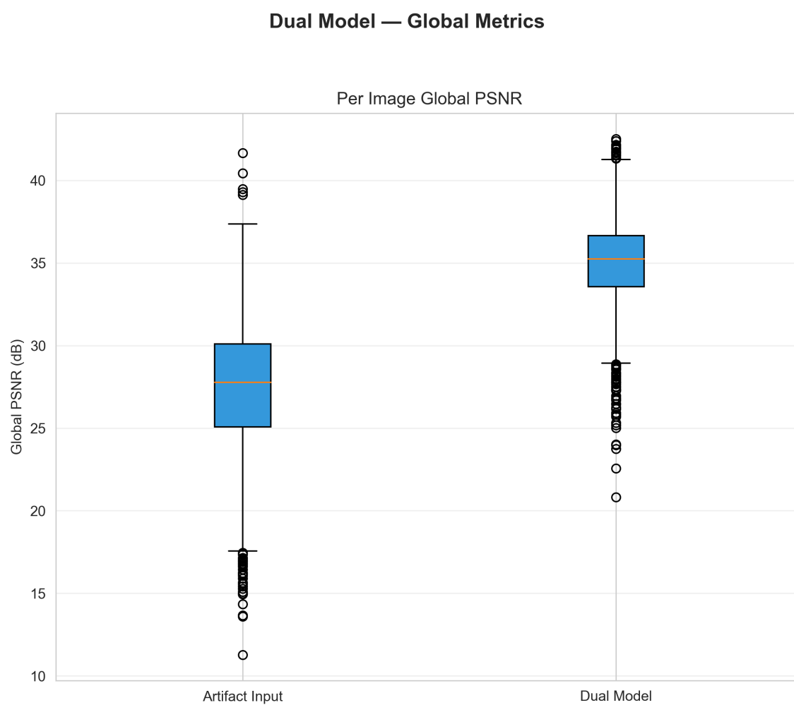
Fig.5.28 Distribuicao de metricas e analise de correlacao: boxplot_global_psnr_distribution.png .
