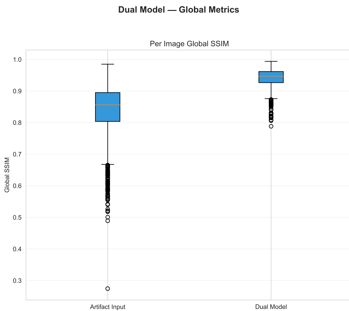
Fig.5.29 Distribuicao de metricas e analise de correlacao: boxplot_global_ssim_distribution.pdf.
