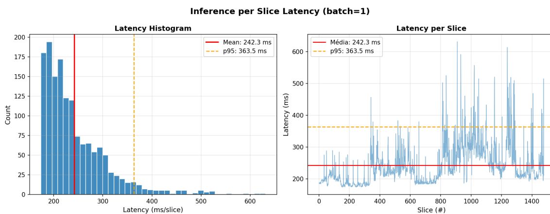
Fig.5.20 Benchmark de inferencia: benchmark_latency.png.
