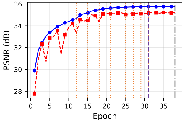
Global PSNR
