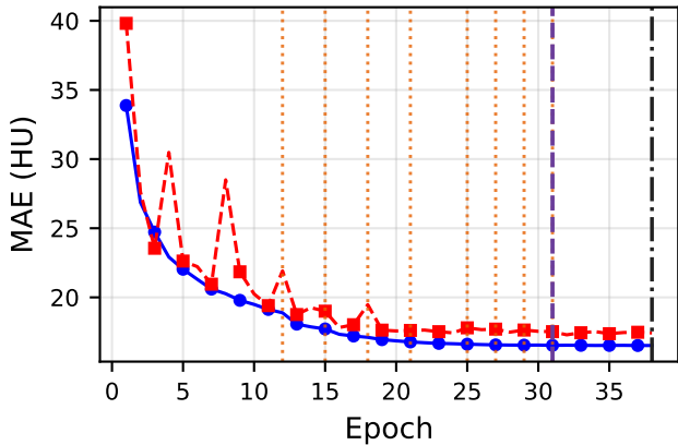
Global MAE
