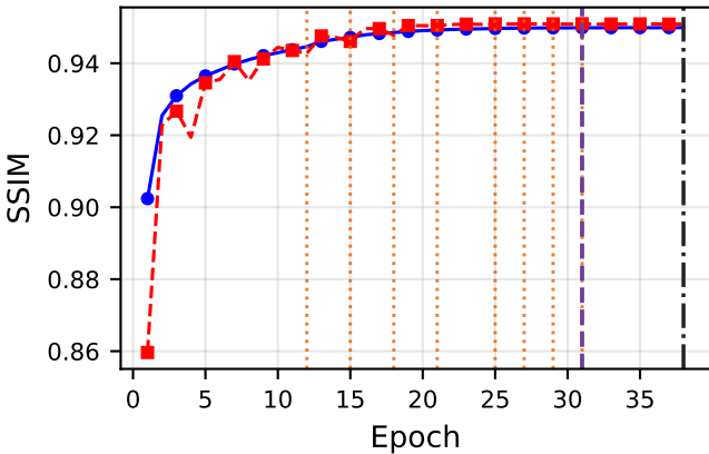
Global SSIM
