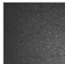
GAPS384
