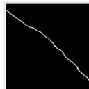
Baseline
