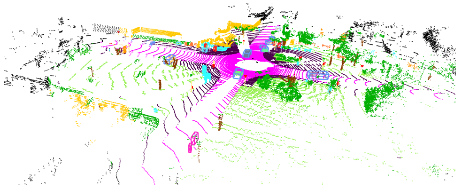
FIGURE 5.4 : Résultat de notre méthode sur la trame 60, séquence o8, de SemanticKITTI. Chaque piste est repérée par sa boîte englobante (une couleur par classe d'objets). Noter les deux cyclistes (boîtes roses) en bas, bien séparés quoique proches (et ce grâce au suivi par transport optimal, quand le clustering avec a priori géométriques les avait fusionnés).
