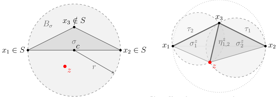
(b) Les K -simplexes \sigma_1^z et \sigma_2^z ont des rayons < r . Le chemin \tau_1 \xrightarrow{\sigma_1^z} \eta_{1,2}^z \xrightarrow{\sigma_2^z} \tau_2 connecte les facettes actives dans \Gamma_K(\mathcal{X})_{<r} .
