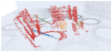
Détection des anomalies (cubes et tuteurs colorés) par rapport au modèle 3D (en rouge) sur le benchmark de Marie ASPRO. © Marie ASPRO / Naval Group.
