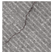
squelette extrait
