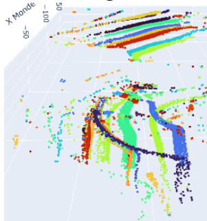
Notre algorithme
