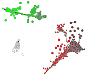
HDBSCAN : 3 macrorégions
