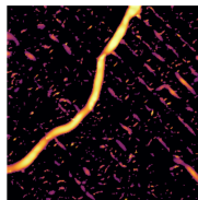
similarité d'arête
