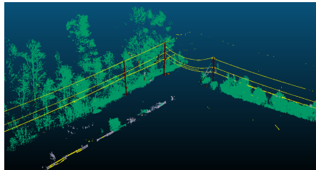
Figure 1 du papier GRETSI (Hydro-Québec) : Nuage LiDAR sans sol et classifié.
