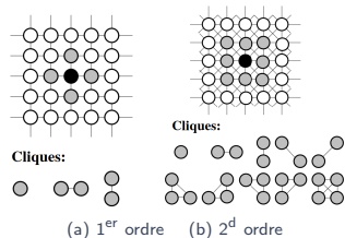
(a) 1 er ordre (b) 2 d ordre Voisinages entre pixels dans une grille et cliques associées [29].
