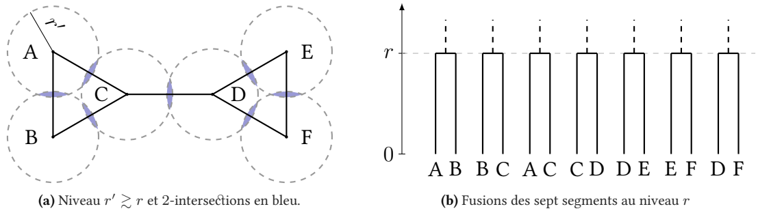
FIGURE 6.2 : (Gauche) Nuage \mathcal{X} repris de la FIG. 6.1a avec les amas (en bleu) de forte densité 2-NN au niveau r' \gtrsim r . (Droite) Hiérarchie en construction. Par convention, le multi-ensemble des feuilles apparaît au niveau 0.
