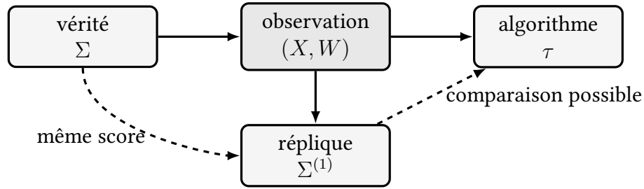
FIGURE 11.5 : La vérité cachée \Sigma peut être remplacée par une réplique postérieure \Sigma^{(1)} . Toute l'astuce de la suite du chapitre consiste à construire \Sigma^{(1)} en faisant un pas d'une dynamique de clusters à partir de \Sigma .
