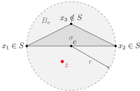
(a) Un triangle \sigma = \{x_1, x_2, x_3\} . B_\sigma a pour diamètre [x_1, x_2] . L'ensemble de support est S = \{x_1, x_2\} . \sigma n'est pas de GABRIEL donc il existe un "intrus" z \in \overset{\circ}{B}_\sigma .
