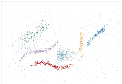
Groupes (HDBSCAN)
