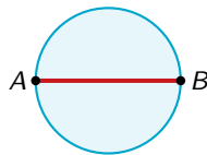
Arête de Gabriel (vide)
