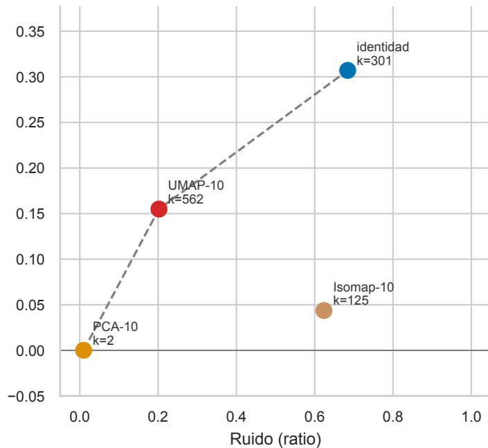
A · Calidad: silueta vs. ruido
