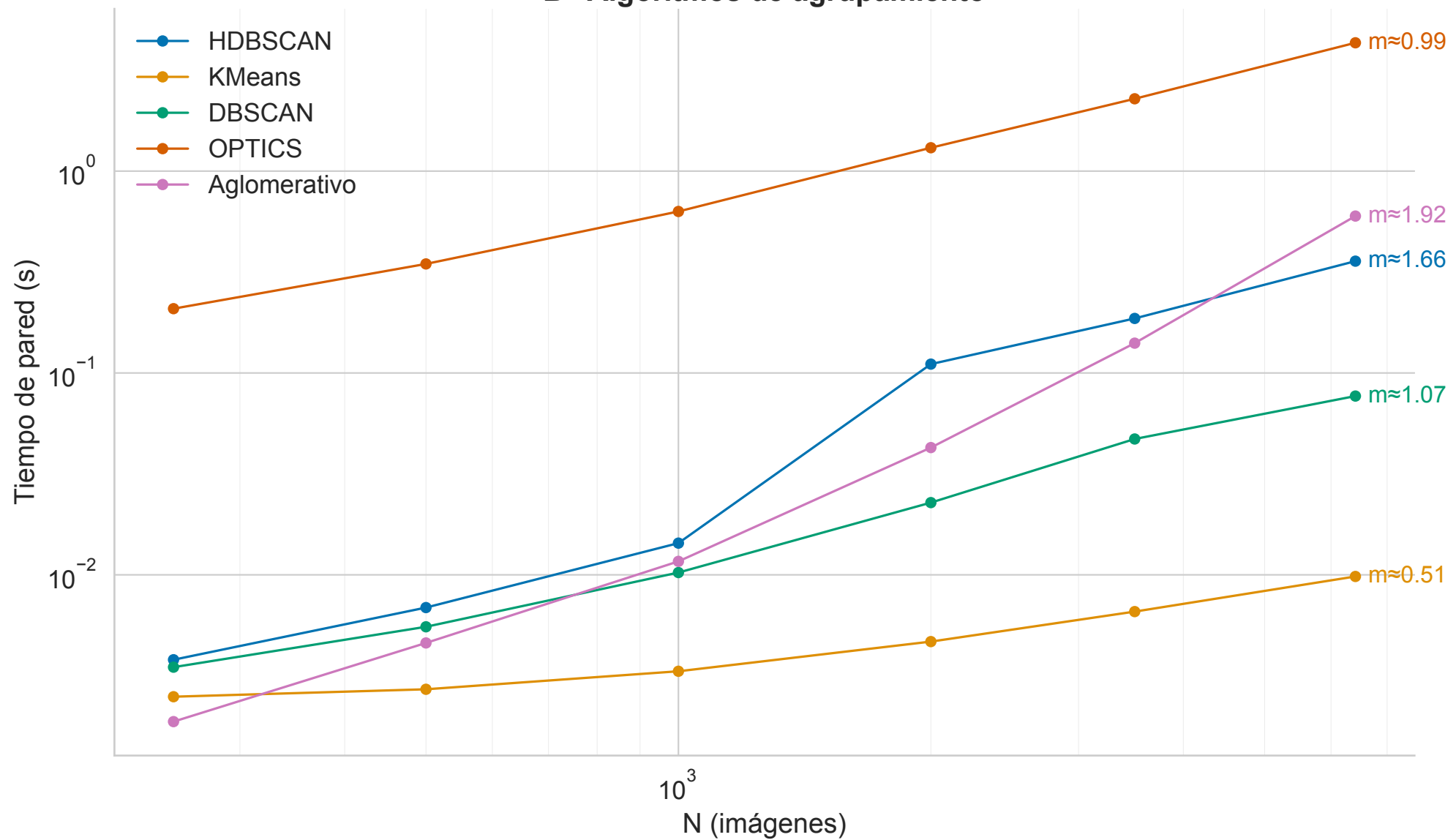
B · Algoritmos de agrupamiento
