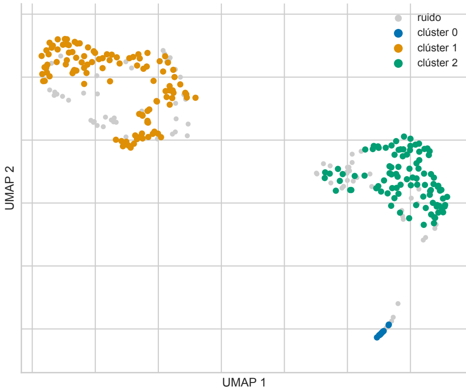
E8a · DINOv2 style-head — clusters HDBSCAN (mcs=5)
